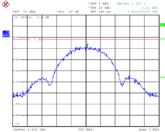
Test Mode : ANT1 Low channel
