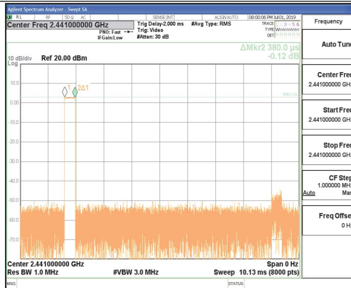
DH1_Ant1_Hop
