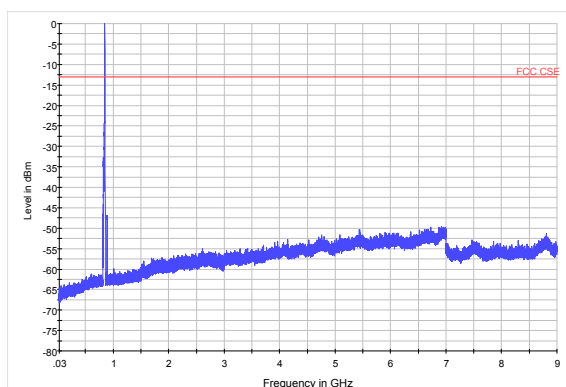
WCDMA Band V CH-High 30MHz ~ 9GHz
