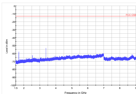
LTE Band 5 5MHz CH-Low 1.5GHz~9GHz
