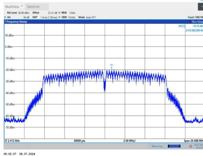
11G_Ant2_2412
