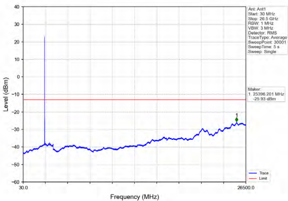
Band38_20MHz_QPSK_LCH_2580MHz_RB_1_0_NTNV
