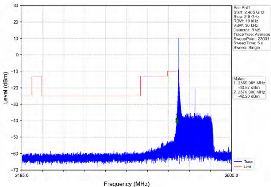
Band38_20MHz_QPSK_LCH_2580MHz_RB_1_0_NTNV
