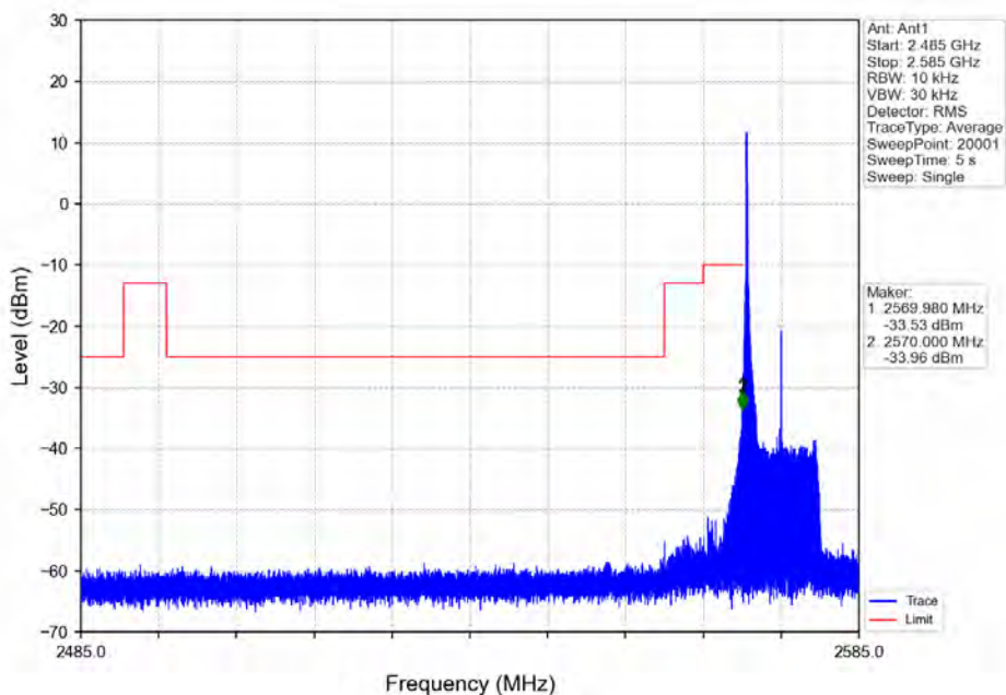
Band38_10MHz_QPSK_LCH_2575MHz_RB_1_0_NTNV
