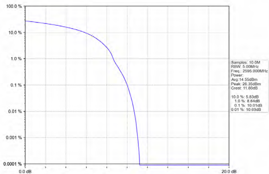
Band38_20MHz_QPSK_MCH_2595MHz_RB_100_0_NTNV
