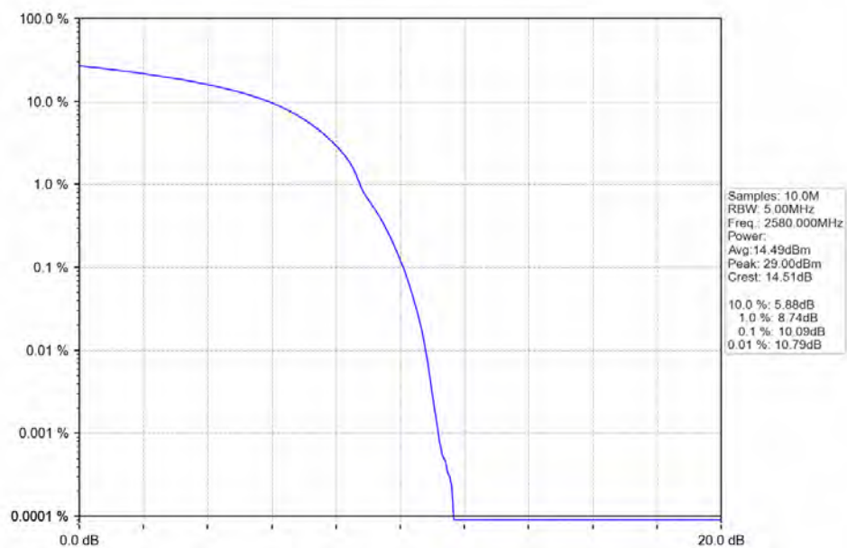
Band38_20MHz_QPSK_LCH_2580MHz_RB_100_0_NTNV
