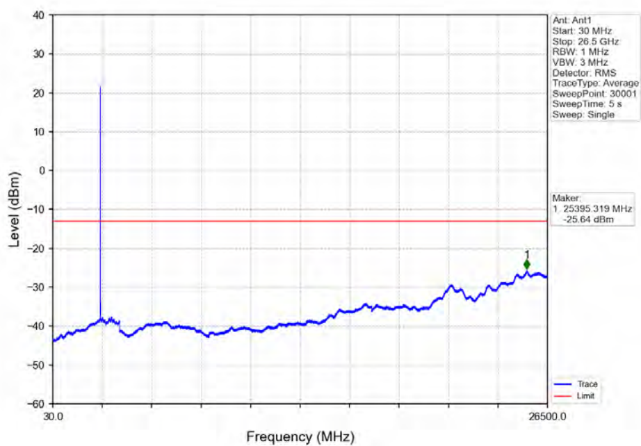
Band38_5MHz_QPSK_LCH_2572.5MHz_RB_1_0_NTNV
