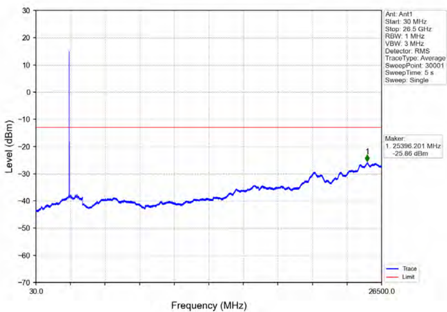
Band38_10MHz_QPSK_LCH_2575MHz_RB_1_0_NTNV
