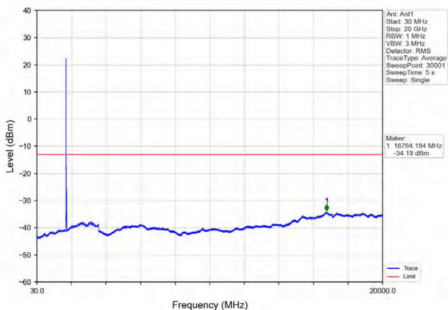
Band4_20MHz_QPSK_LCH_1720MHz_RB_1_0_NTNV
