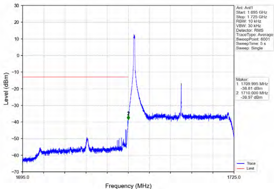
Band4_15MHz_QPSK_LCH_1717.5MHz_RB_1_0_NTNV
