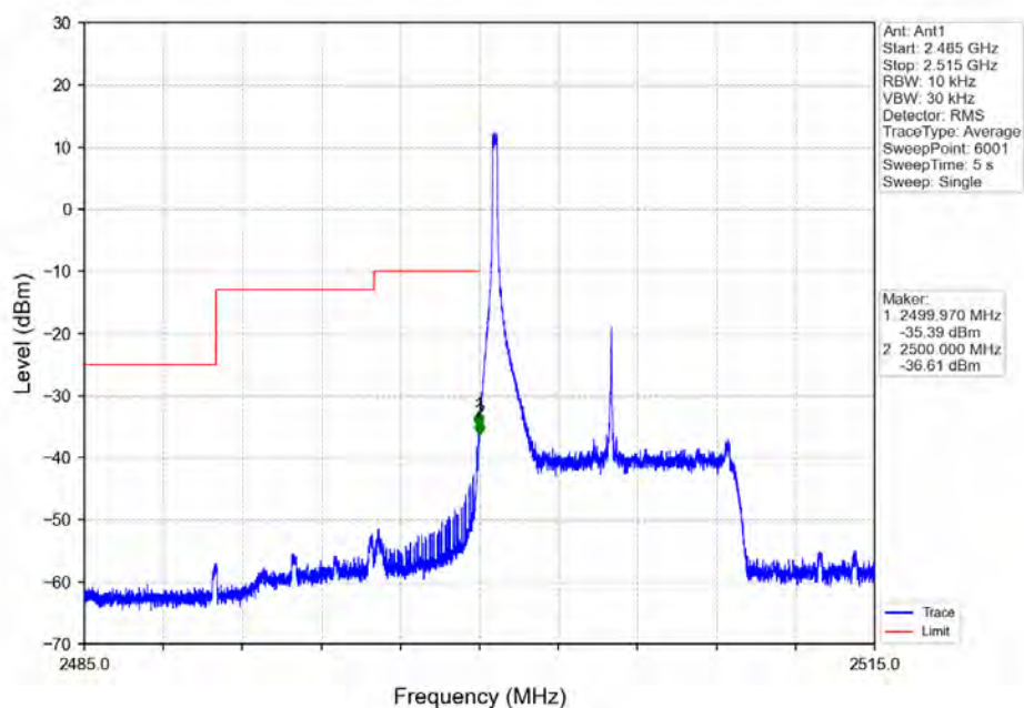
Band7_10MHz_QPSK_LCH_2505MHz_RB_1_0_NTNV
