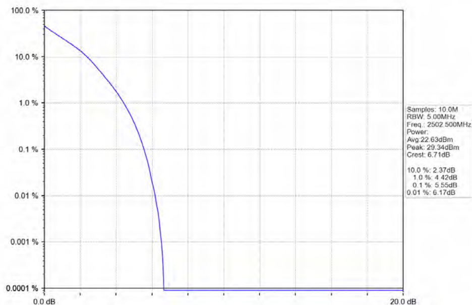
Band7_5MHz_QPSK_LCH_2502.5MHz_RB_25_0_NTNV
