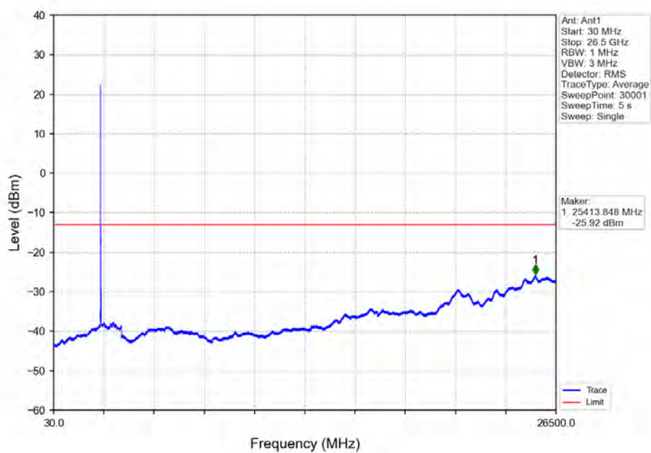
Band7_20MHz_QPSK_LCH_2510MHz_RB_1_0_NTNV
