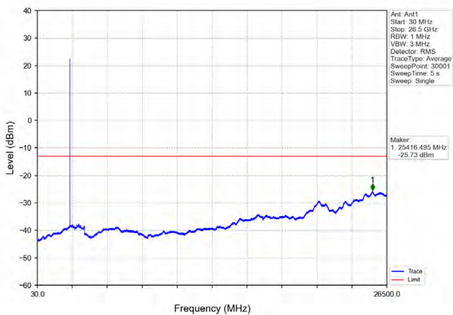
Band7_5MHz_QPSK_LCH_2502.5MHz_RB_1_0_NTNV
