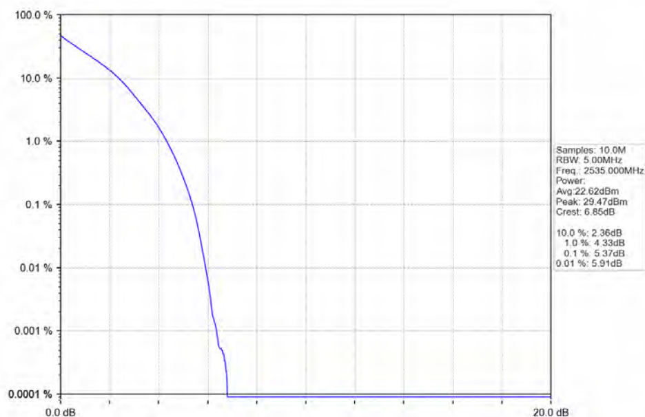
Band7_5MHz_QPSK_MCH_2535MHz_RB_25_0_NTNV
