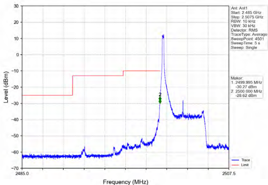
Band7_5MHz_QPSK_LCH_2502.5MHz_RB_1_0_NTNV
