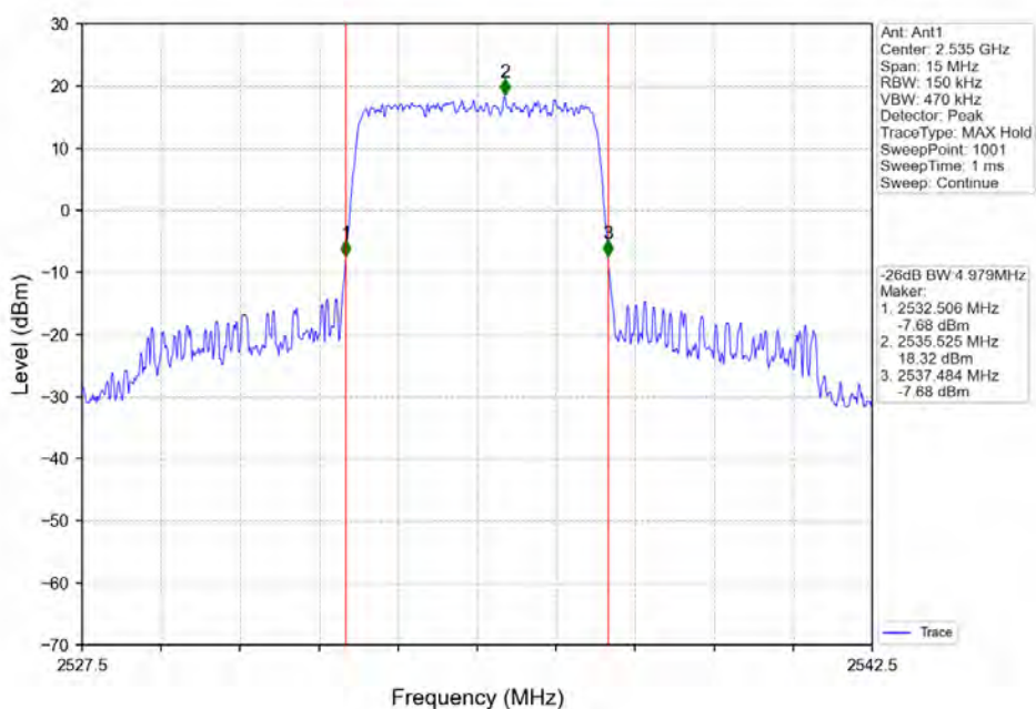
Band7_5MHz_QPSK_MCH_2535MHz_RB_25_0_NTNV
