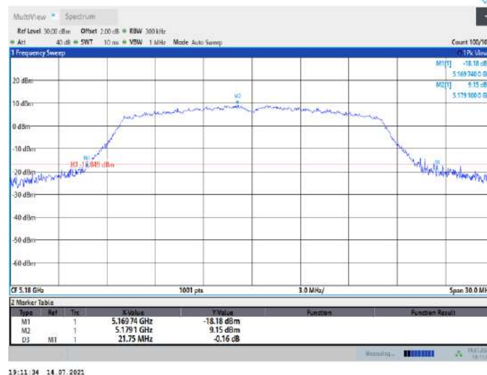
11A Ant9 5180
