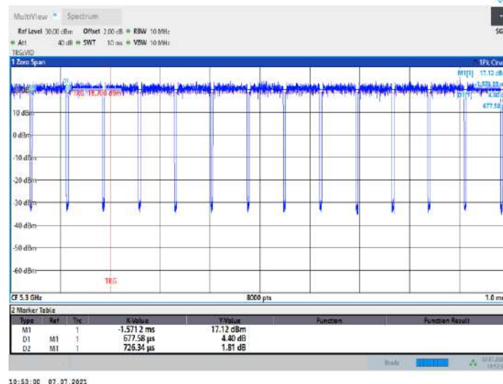
11AC20MIMO_Ant9_5300
