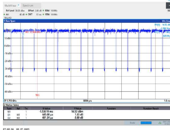
11N40MIMO_Ant9_5755
