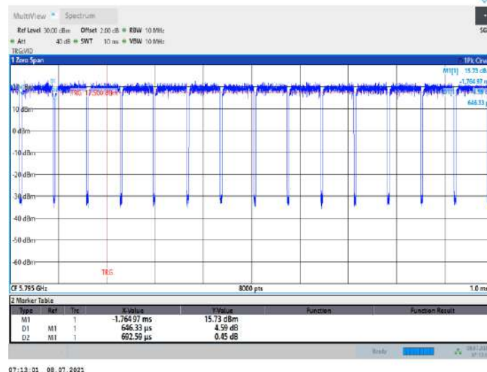
11N40MIMO_Ant9_5795
