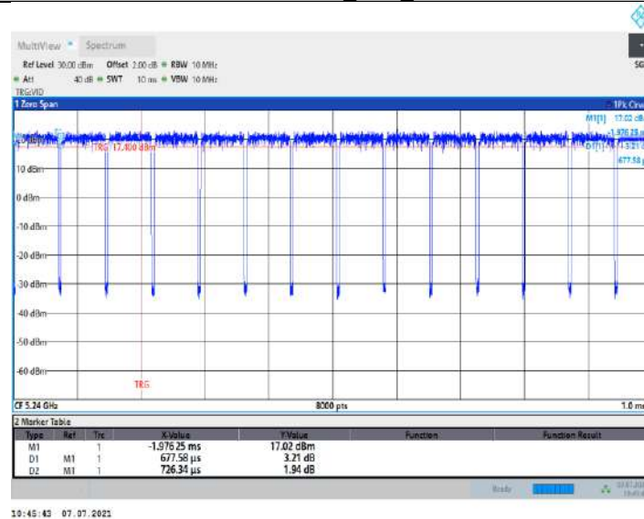
11AC20MIMO_Ant9_5240
