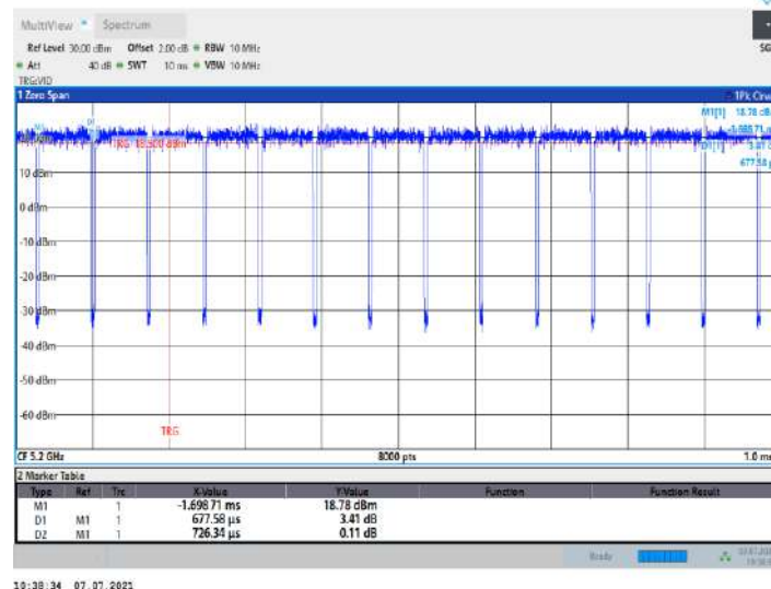
11AC20MIMO_Ant9_5200
