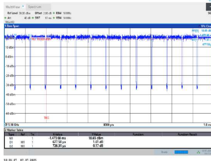
11AC20MIMO_Ant9_5180
