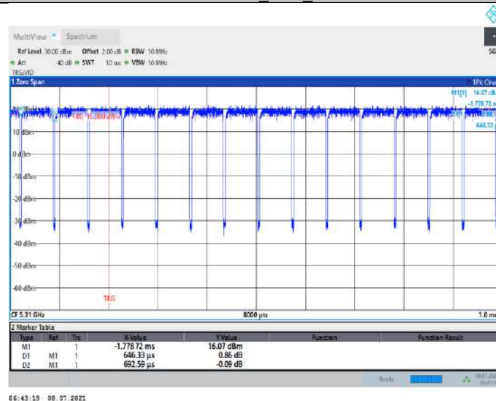
11N40MIMO_Ant9_5310
