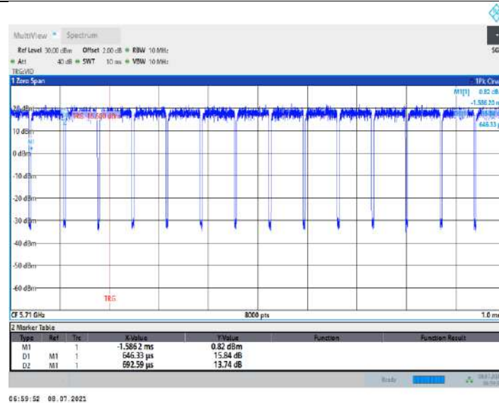
11N40MIMO_Ant9_5710
