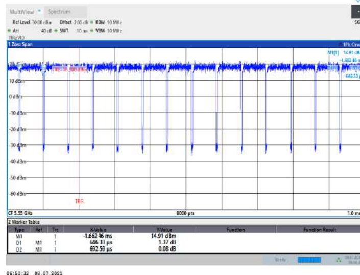
11N40MIMO_Ant9_5550
