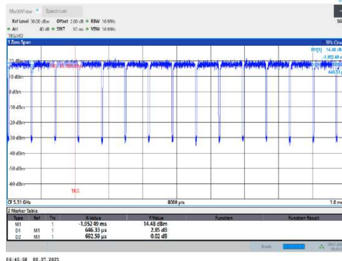
11N40MIMO_Ant9_5510
