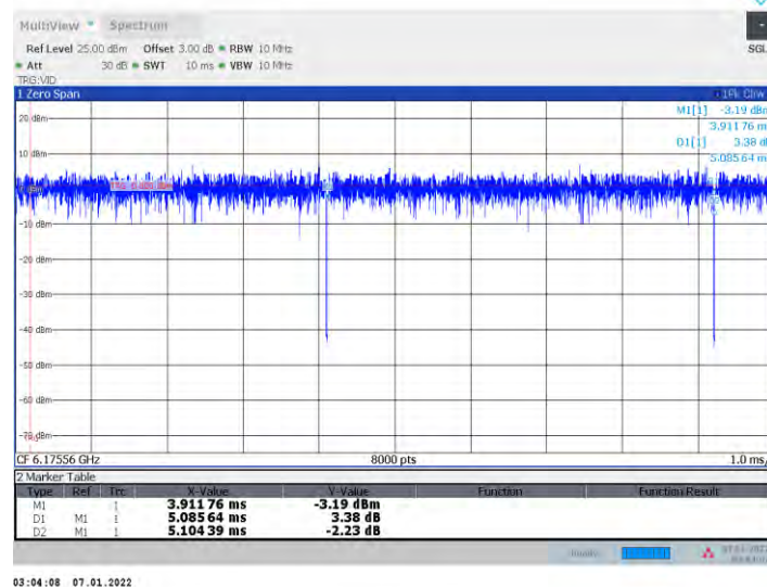
11AX20MIMO_Ant1_6175_52Tone_RU38
