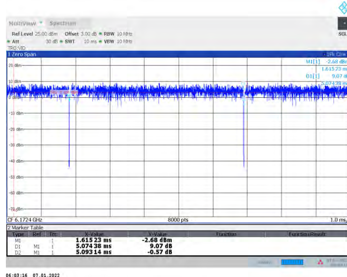
11AX20MIMO_Ant1_6175_52Tone_RU38
