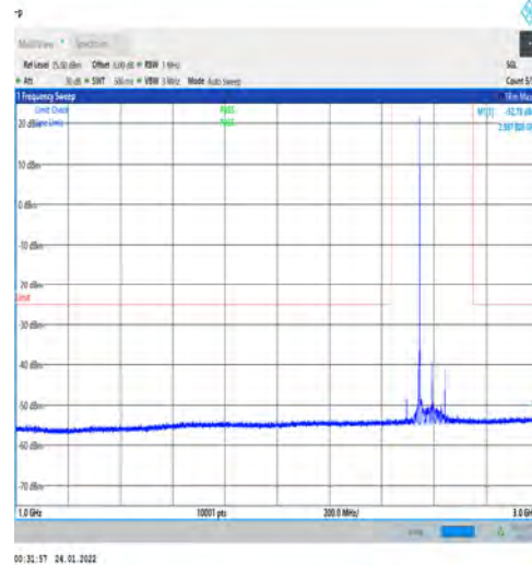
1-N41-PC3-30-100-M-1-DFT-PI2BPSK-Edge_1RB_L eft-1@0-1000-3000-Ant1--52.78--25-PASS
