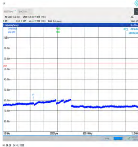
1-N41-PC3-30-100-L-1-DFT-PI2BPSK-Edge_1RB_L eft-1@0-3000-12000-Ant1--58.10--25-PASS
