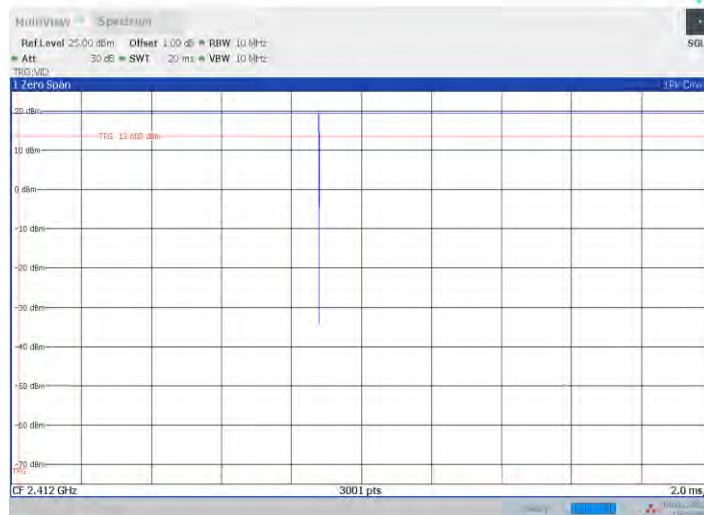
11B-CDD_Ant17_2412
