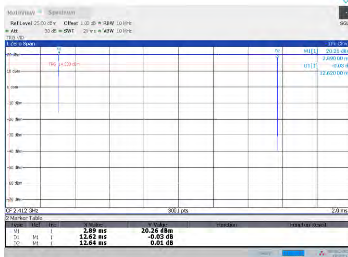
11B-CDD_Ant17_2412
