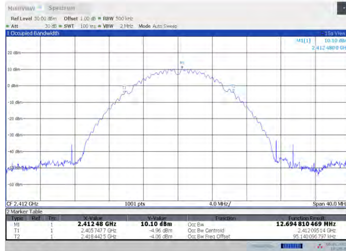
11B-CDD_Ant17_2412
