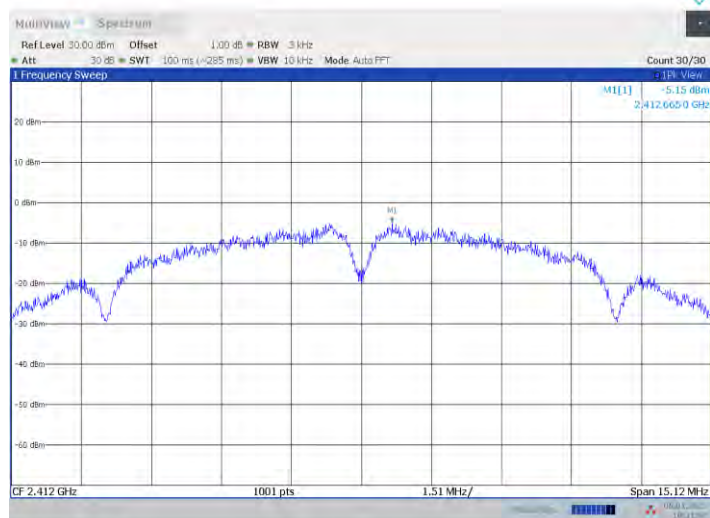
11B-CDD_Ant17_2412
