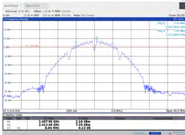
11B-CDD_Ant17_2412
