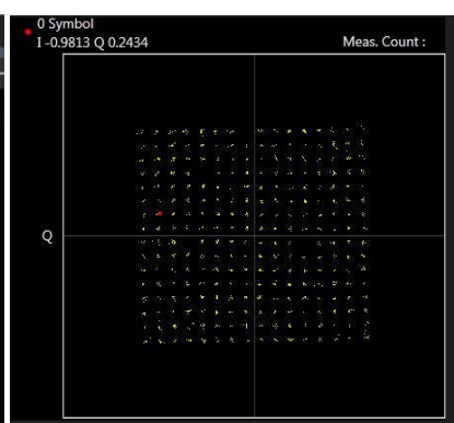
256QAM
