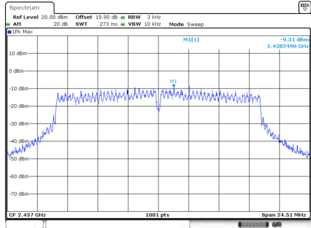
MIMO Ant. 18
