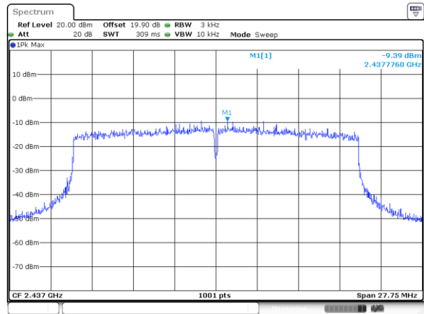
MIMO Ant. 18
