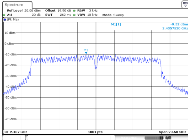
MIMO Ant. 16
