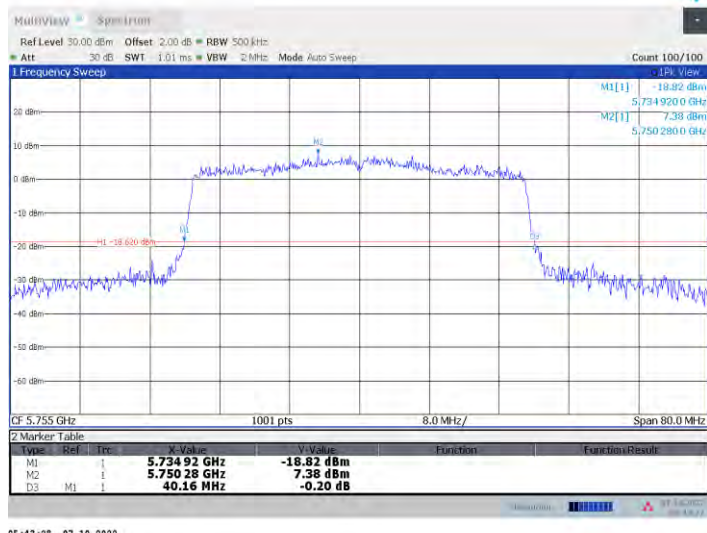
11ax40MIMO_Ant8_5755
