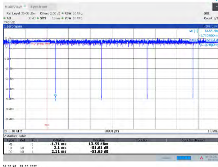
11a-CDD_Ant8_5180
