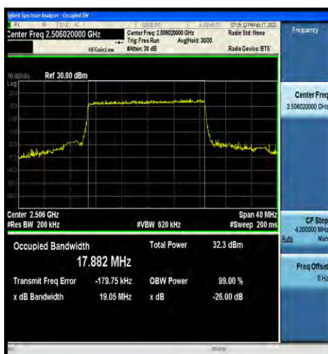
1-N41-30-20-L-3-DFT-16QAM-Outer_Full-50@0-Ant 2-17.882-19.05-≤20-PASS
