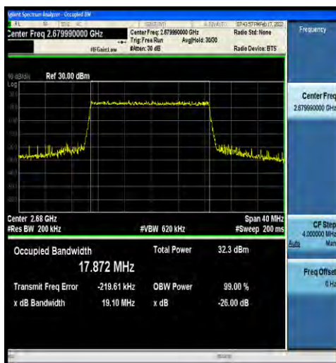
1-N41-30-20-H-3-DFT-16QAM-Outer_Full-50@0-Ant 2-17.872-19.10-≤20-PASS
