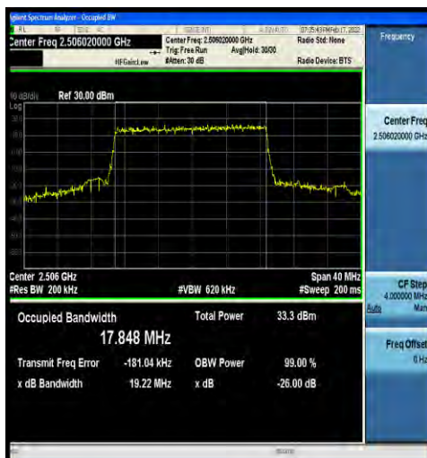
1-N41-30-20-L-1-DFT-QPSK-Outer_Full-50@0-Ant2- 17.848-19.22-≤20-PASS
