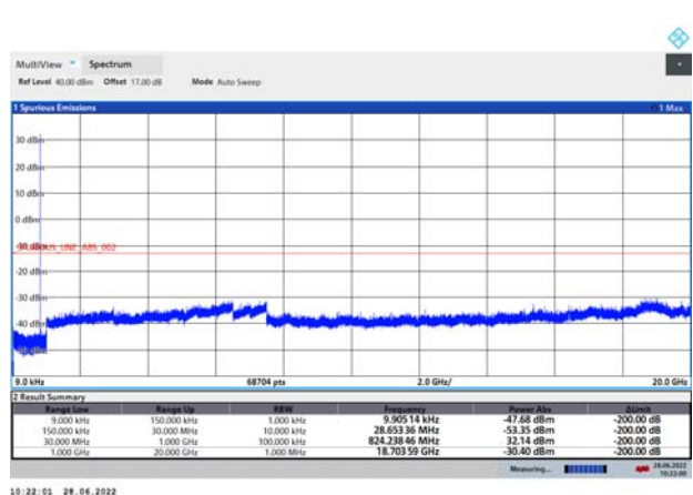
GSM 850 CH-Middle 9kHz ~ 20GHz
