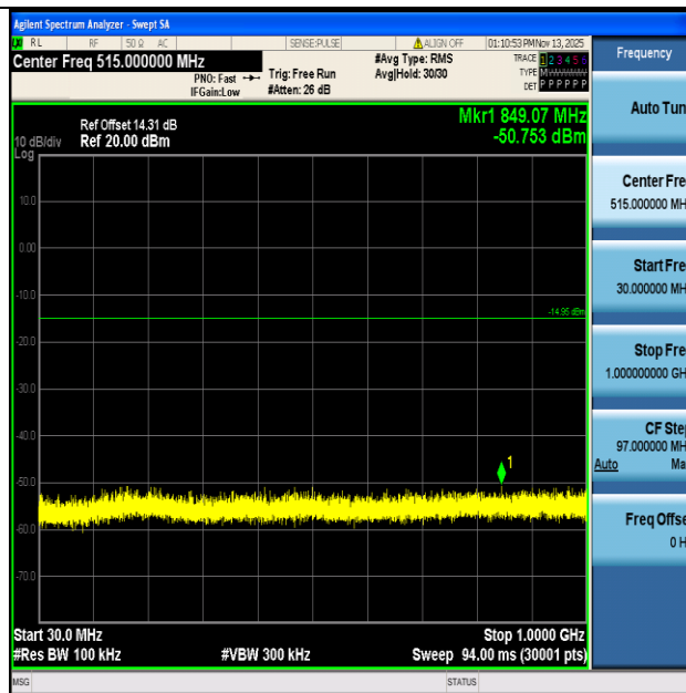
BLE_2M-Ant1-2480-30~1000-PASS
