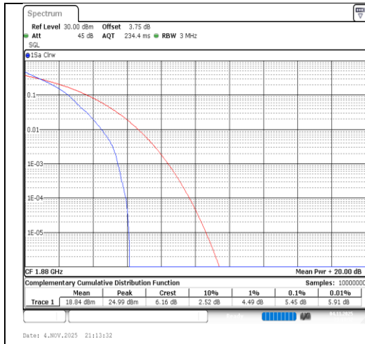
Band2-3MHz-QPSK-18900-1RB#0-PASS
