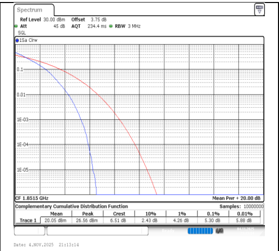
Band2-3MHz-QPSK-18615-15RB#0-PASS
