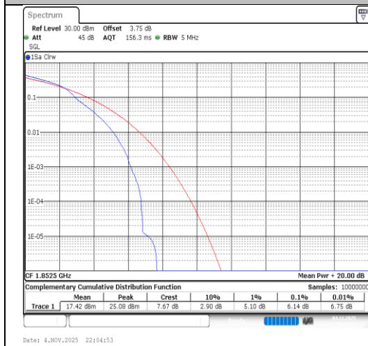
Band2-5MHz-16QAM-18625-1RB#0-PASS
