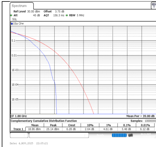
Band2-5MHz-QPSK-18900-1RB#0-PASS
