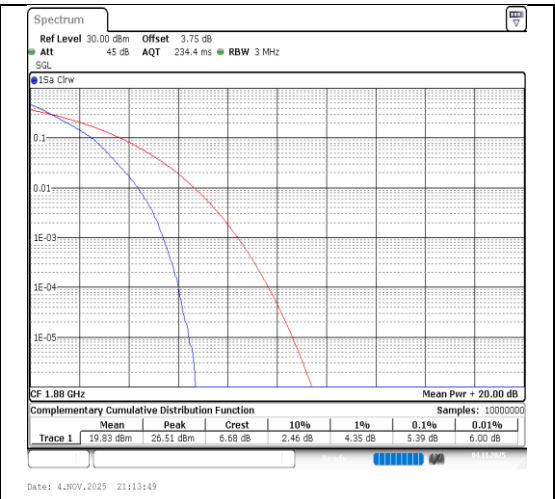
Band2-3MHz-QPSK-18900-15RB#0-PASS
