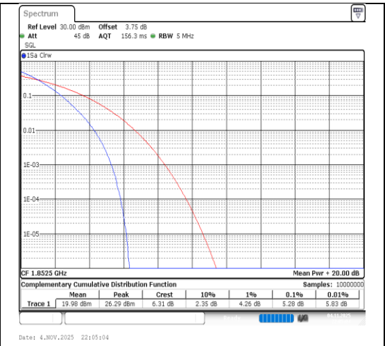
Band2-5MHz-QPSK-18625-25RB#0-PASS
