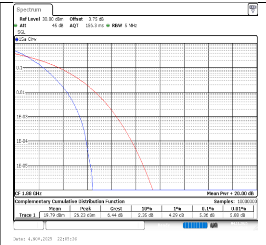
Band2-5MHz-QPSK-18900-25RB#0-PASS
