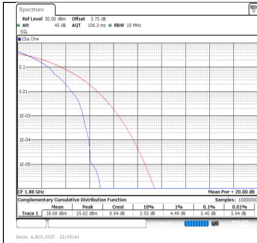
Band2-10MHz-QPSK-18900-1RB#0-PASS
