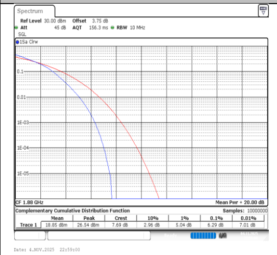
Band2-10MHz-16QAM-18900-50RB#0-PASS
