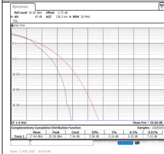
Band2-20MHz-16QAM-19100-1RB#0-PASS
