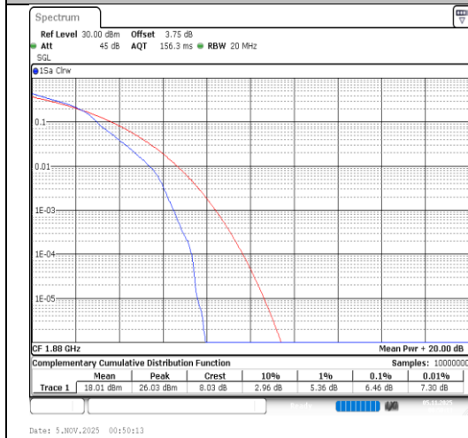
Band2-20MHz-16QAM-18900-1RB#0-PASS
