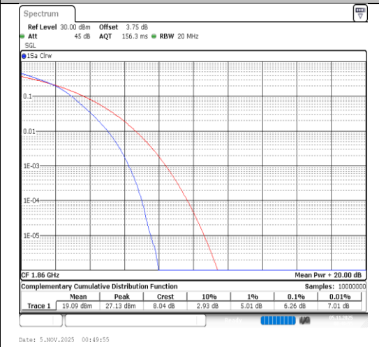
Band2-20MHz-16QAM-18700-100RB#0-PASS
