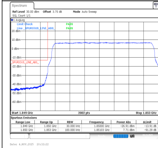
Band2-3MHz-QPSK-18615-15RB#0-PASS
