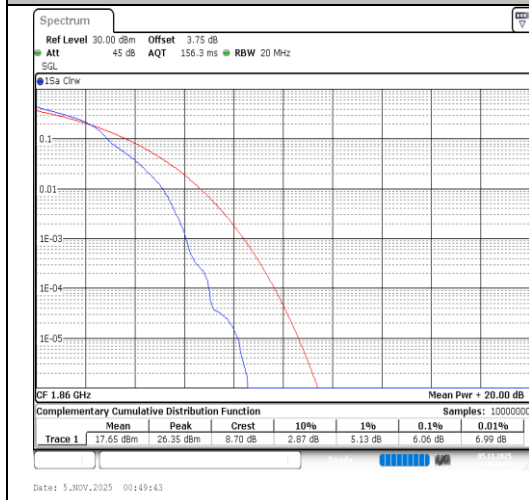
Band2-20MHz-64QAM-18700-1RB#0-PASS
