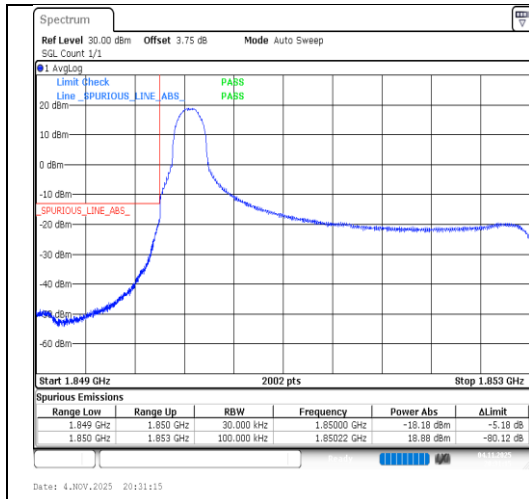
Band2-3MHz-QPSK-18615-1RB#0-PASS
