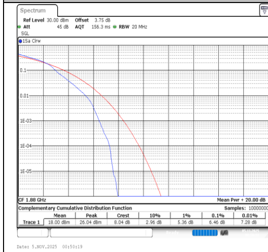
Band2-20MHz-64QAM-18900-1RB#0-PASS
