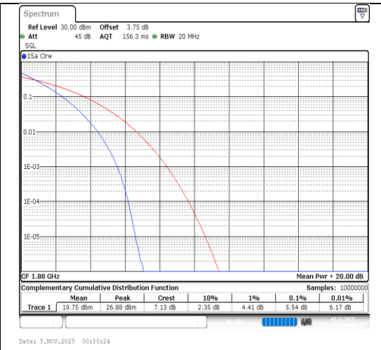
Band2-20MHz-QPSK-18900-100RB#0-PASS
