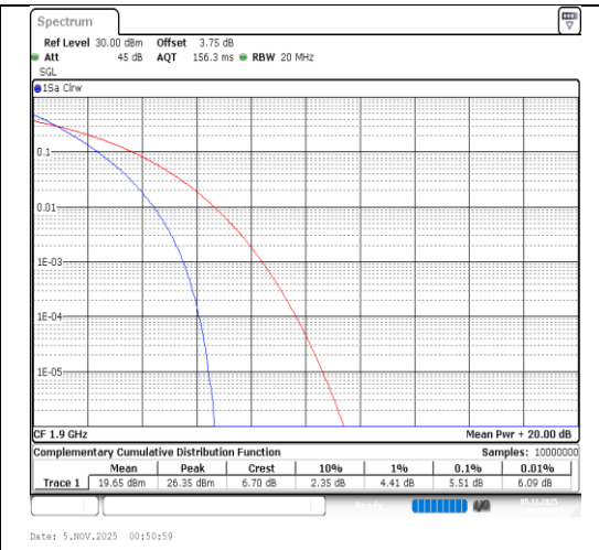
Band2-20MHz-QPSK-19100-100RB#0-PASS
