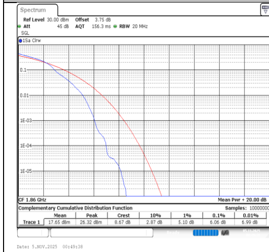
Band2-20MHz-16QAM-18700-1RB#0-PASS
