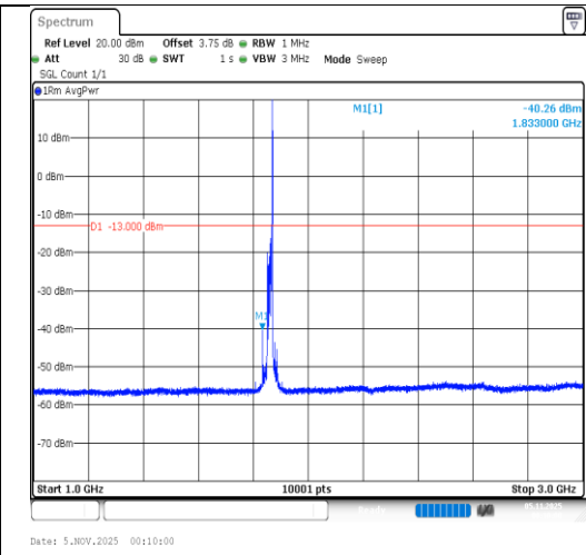
Band2-20MHz-QPSK-18700-1RB#99-1000~3000-PASS
