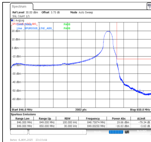
Band26(824-849)-3MHz-QPSK-27025-1RB#14-PASS
