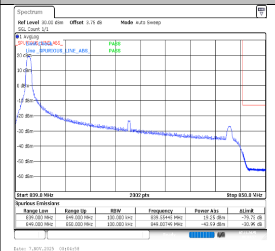
Band26(824-849)-10MHz-QPSK-26990-1RB#0-PASS
