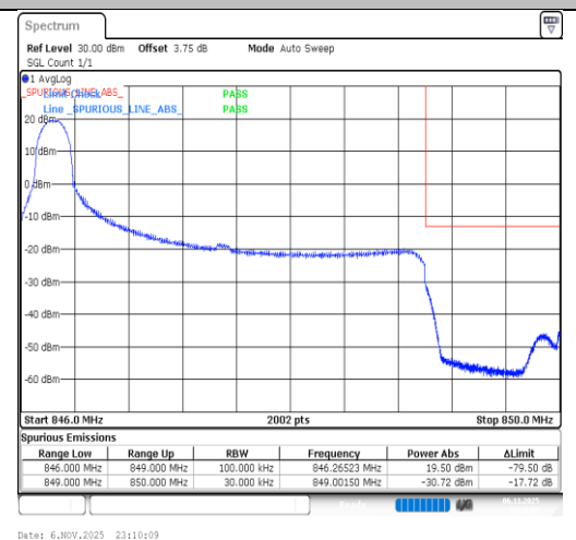
Band26(824-849)-3MHz-QPSK-27025-1RB#0-PASS
