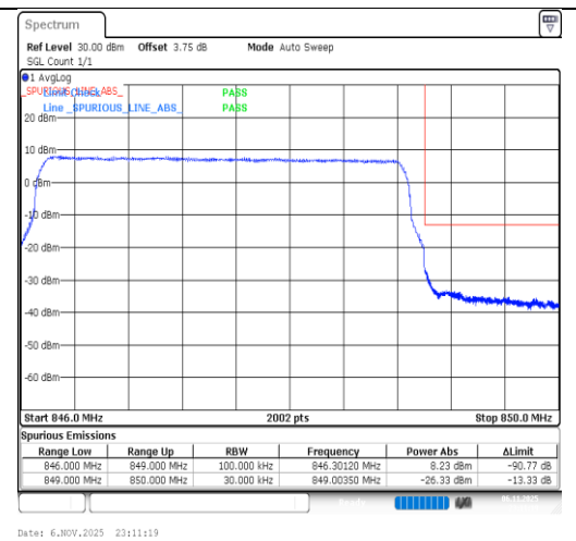
Band26(824-849)-3MHz-QPSK-27025-15RB#0-PASS
