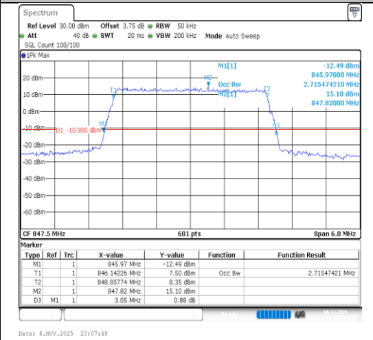
Band26(824-849)-3MHz-QPSK-27025-15RB#0-PASS
