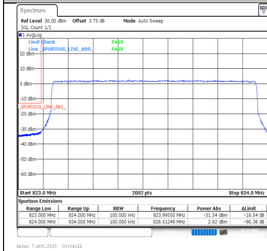
Band26(824-849)-10MHz-QPSK-26840-50RB#0-PASS
