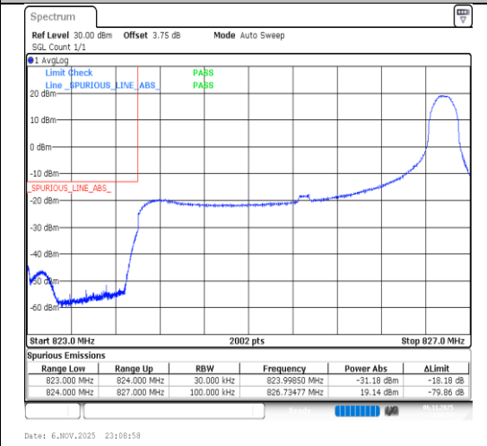
Band26(824-849)-3MHz-QPSK-26805-1RB#14-PASS
