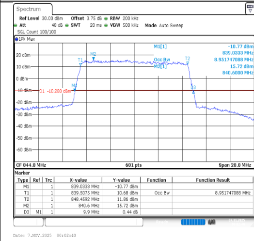
Band26(824-849)-10MHz-QPSK-26990-50RB#0-PASS
