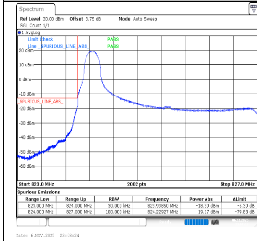
Band26(824-849)-3MHz-QPSK-26805-1RB#0-PASS
