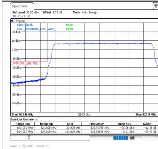
Band26(824-849)-3MHz-QPSK-26805-15RB#0-PASS
