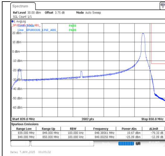
Band26(824-849)-10MHz-QPSK-26990-1RB#49-PASS
