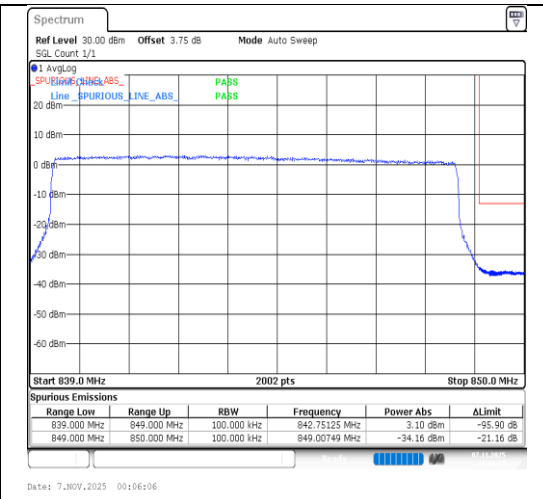
Band26(824-849)-10MHz-QPSK-26990-50RB#0-PASS
