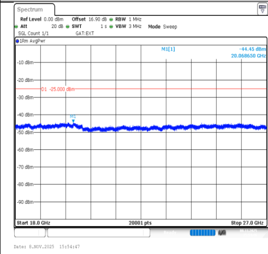
Band38-15MHz-64QAM-37825-1RB#74- 18000~27000-PASS
