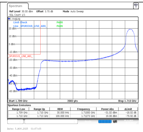
Band4-3MHz-QPSK-19965-1RB#14-PASS
