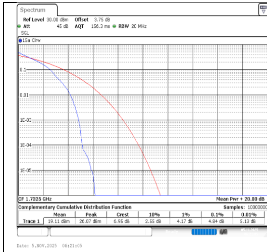
Band4-20MHz-QPSK-20175-1RB#0-PASS
