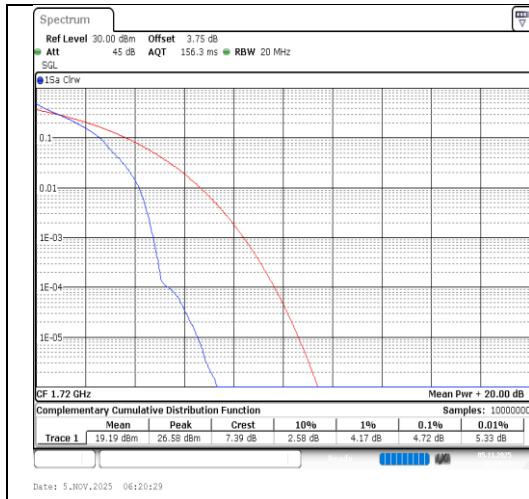
Band4-20MHz-QPSK-20050-1RB#0-PASS
