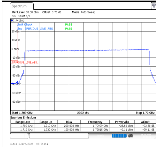
Band4-20MHz-QPSK-20050-100RB#0-PASS
