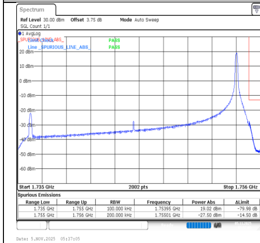
Band4-20MHz-QPSK-20300-1RB#99-PASS
