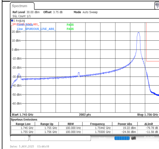
Band4-10MHz-QPSK-20350-1RB#49-PASS
