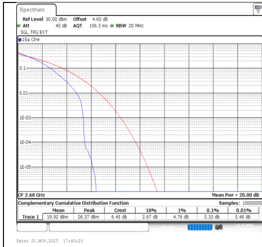
Band41-20MHz-QPSK-41490-1RB#0-PASS
