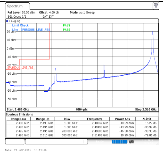
Band41-20MHz-QPSK-39750-1RB#99-PASS
