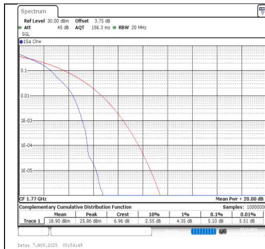
Band66-20MHz-QPSK-132572-1RB#0-PASS
