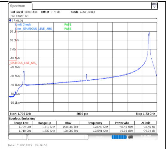
Band66-20MHz-QPSK-132072-1RB#99-PASS
