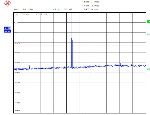
GSM 1900 CH-Middle 1GHz~3GHz
