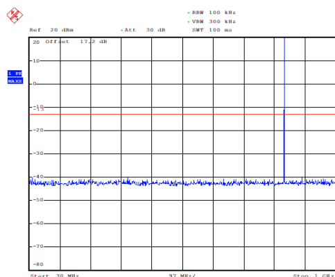
GSM 850 CH-Middle 30MHz ~ 1GHz
