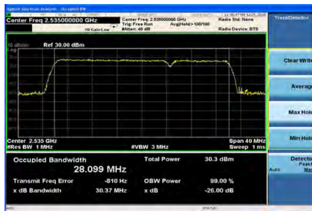
CA-7C 16QAM 20MHz+10MHz
