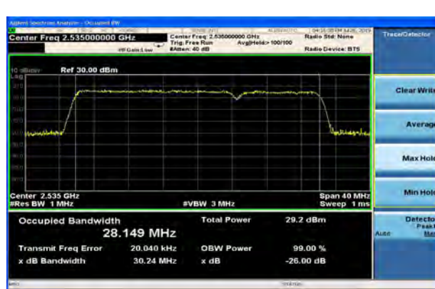
CA-7C 64QAM 20MHz+10MHz
