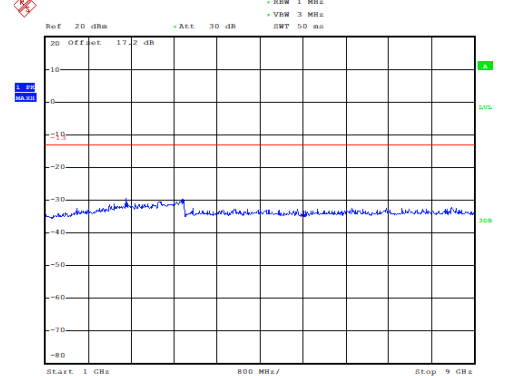
GSM 850 CH-High 1GHz ~ 9GHz
