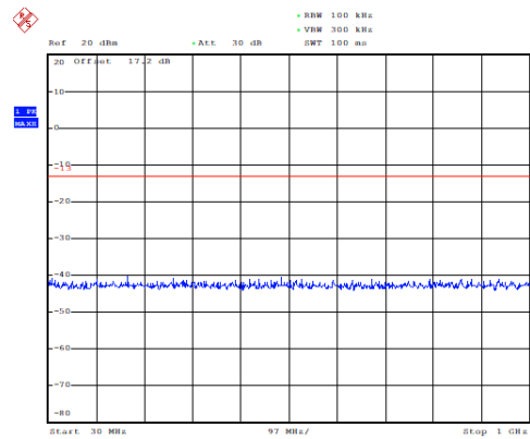
GSM 1900 CH-Middle 30MHz~1GHz
