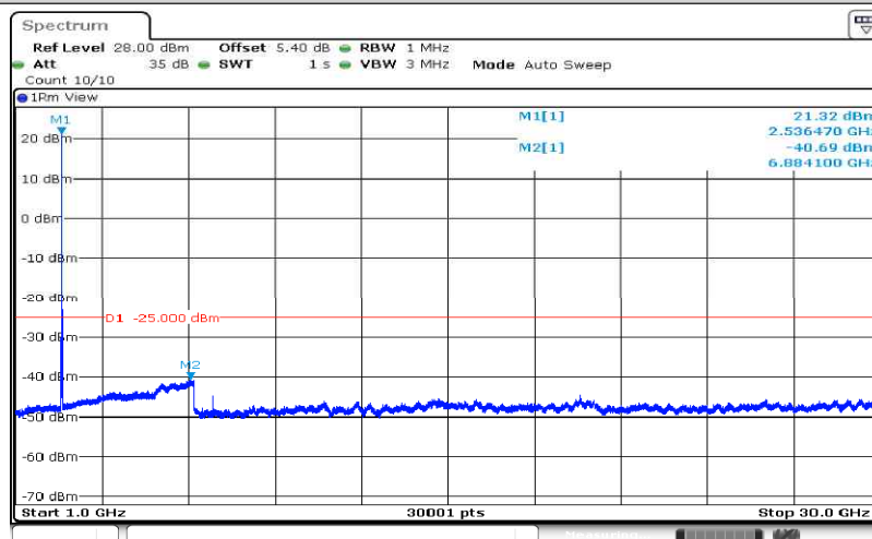
Band41-20MHz-QPSK-40140-1RB#0-Range2:1000~30000MHz
