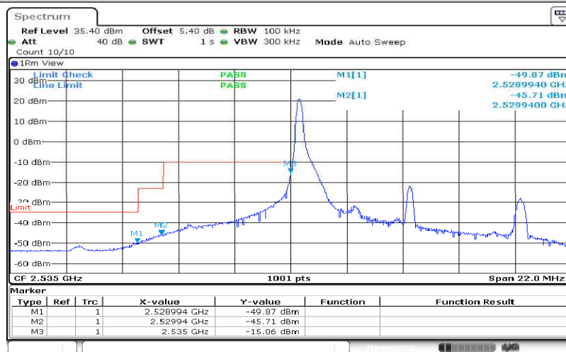
Band41-5MHz-QPSK-40065-1RB#0
