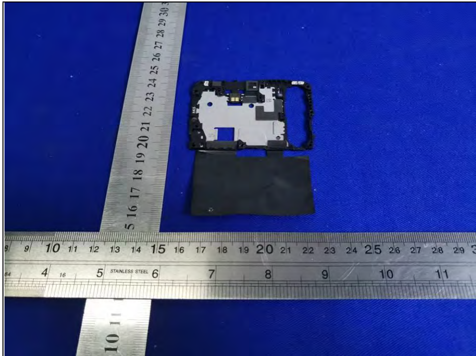
NFC Antenna
