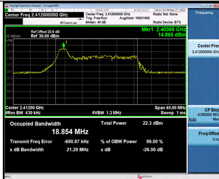
11AX20MIMO_Ant1_2412_52Tone_RU37
