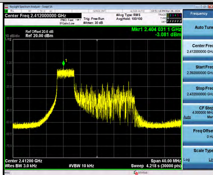
11AX20MIMO_Ant1_2412_106Tone_RU53
