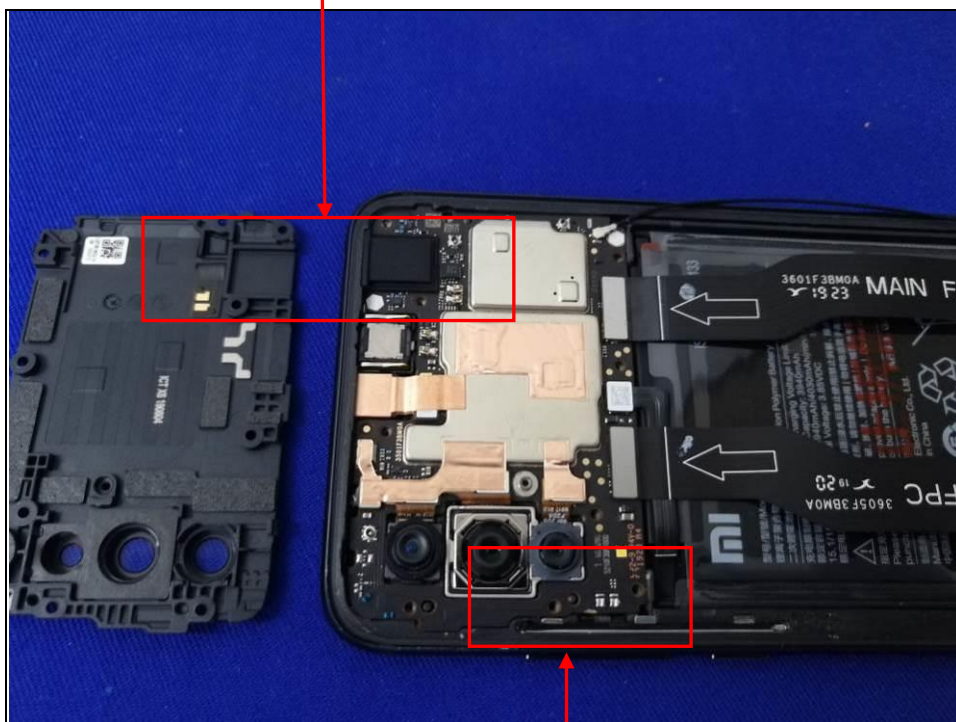
BT/WIFI/GPS Antenna
