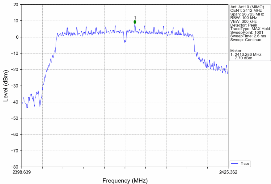
802.11n(HT20)_LCH_2412MHz_Ant10 (MIMO)_NTNV
