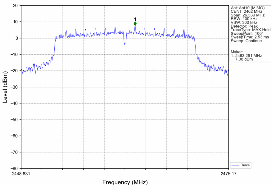
802.11n(HT20)_HCH_2462MHz_Ant10 (MIMO)_NTNV
