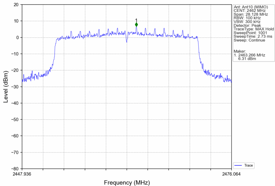
802.11ax(HEW20)_HCH_2462MHz_RU242_Left_Ant10 (MIMO)_NTNV
