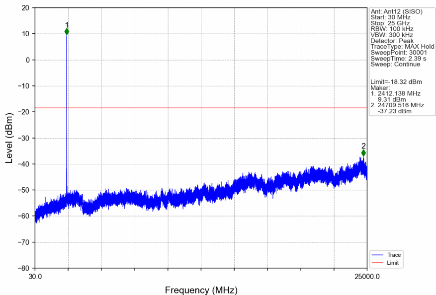
802.11b_LCH_2412MHz_Ant12 (SISO)_NTNV
