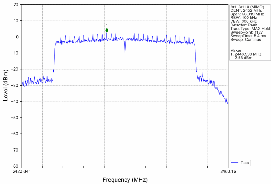
802.11ax(HEW40)_HCH_2452MHz_RU484_Left_Ant10 (MIMO)_NTNV
