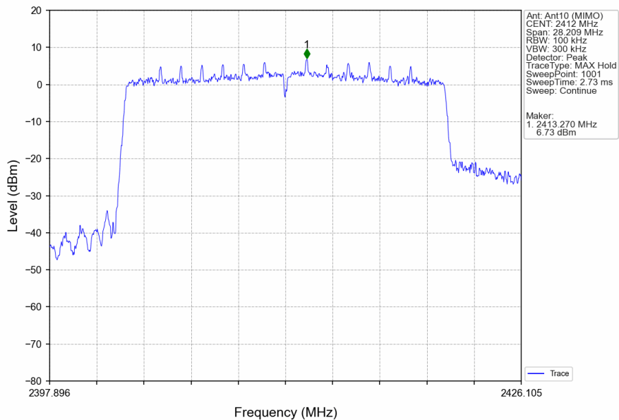
802.11ax(HEW20)_LCH_2412MHz_RU242_Left_Ant10 (MIMO)_NTNV
