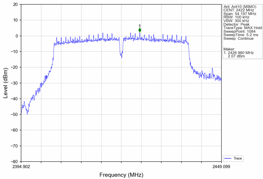
802.11n(HT40)_LCH_2422MHz_Ant10 (MIMO)_NTNV
