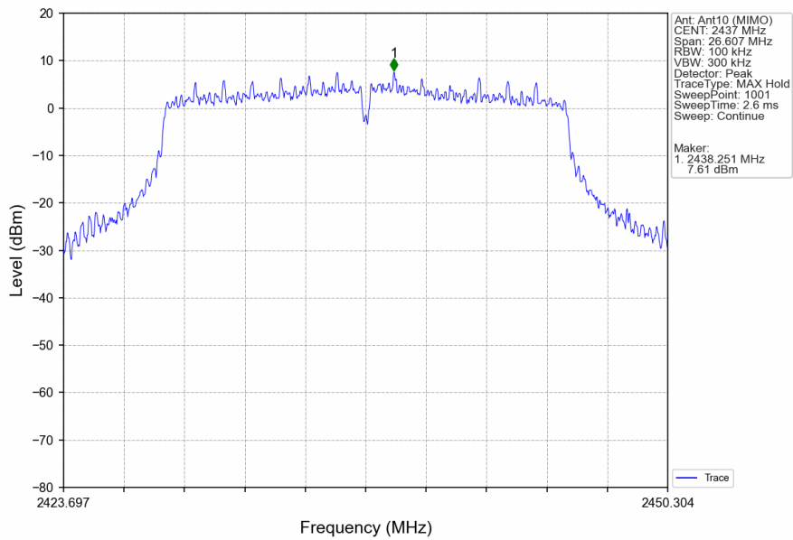
802.11n(HT20)_MCH_2437MHz_Ant10 (MIMO)_NTNV
