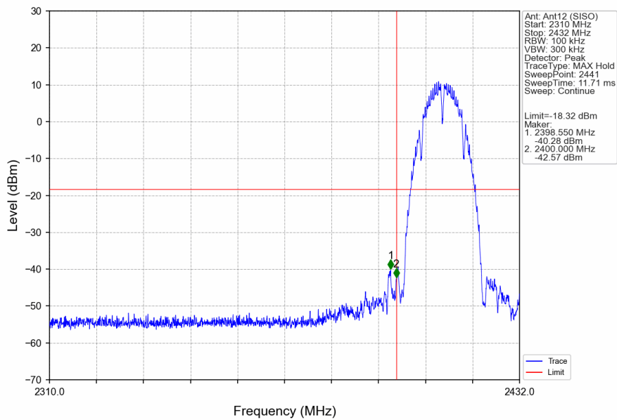
802.11b_LCH_2412MHz_Ant12 (SISO)_NTNV
