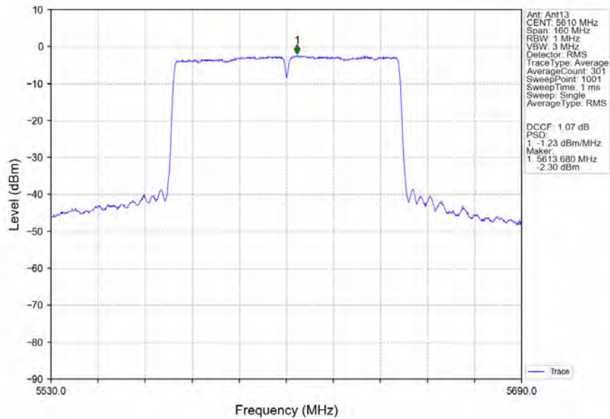
802.11ac(VHT80)_HCH_5610MHz_MIMO_NTNV
