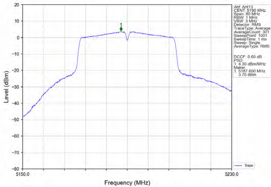
802.11n(HT40)_LCH_5190MHz_Ant13_NTNV
