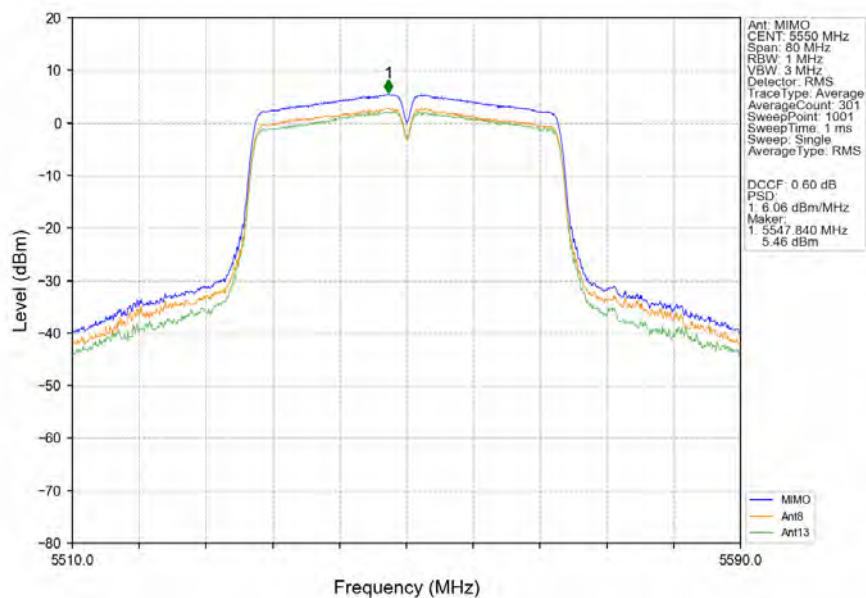
802.11n(HT40)_MCH_5550MHz_MIMO_NTNV
