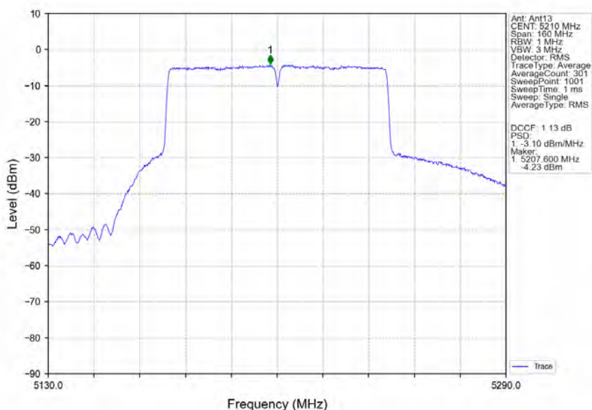
802.11ac(VHT80)_MCH_5210MHz_Ant13_NTNV
