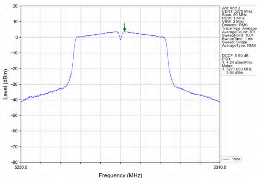
802.11ac(VHT40)_LCH_5270MHz_Ant13_NTNV
