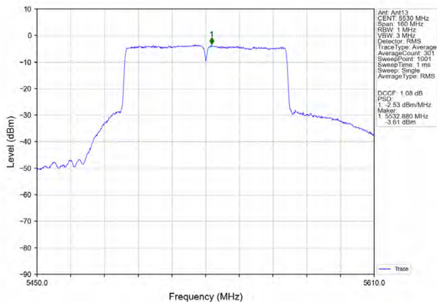
802.11ac(VHT80)_LCH_5530MHz_Ant13_NTNV
