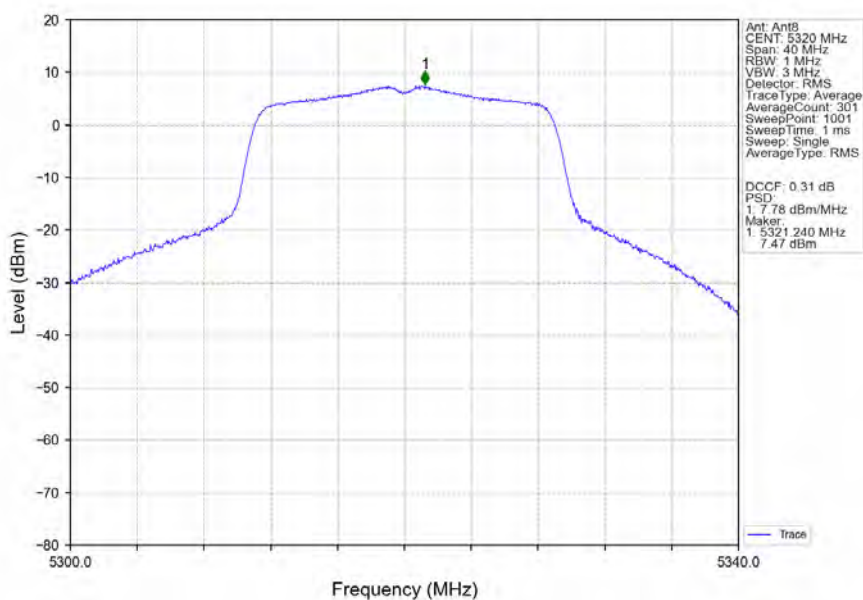
802.11ac(VHT20)_HCH_5320MHz_Ant8_NTNV
