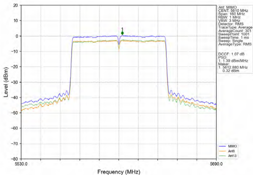
802.11ac(VHT80)_HCH_5610MHz_MIMO_NTNV
