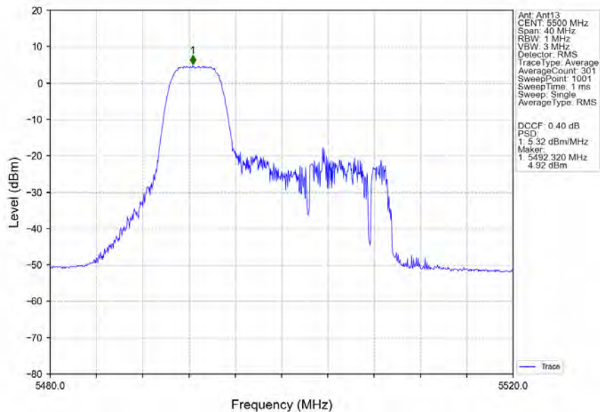
802.11ax(HEW20)_LCH_5500MHz_RU52_Left_Ant13_NTNV
