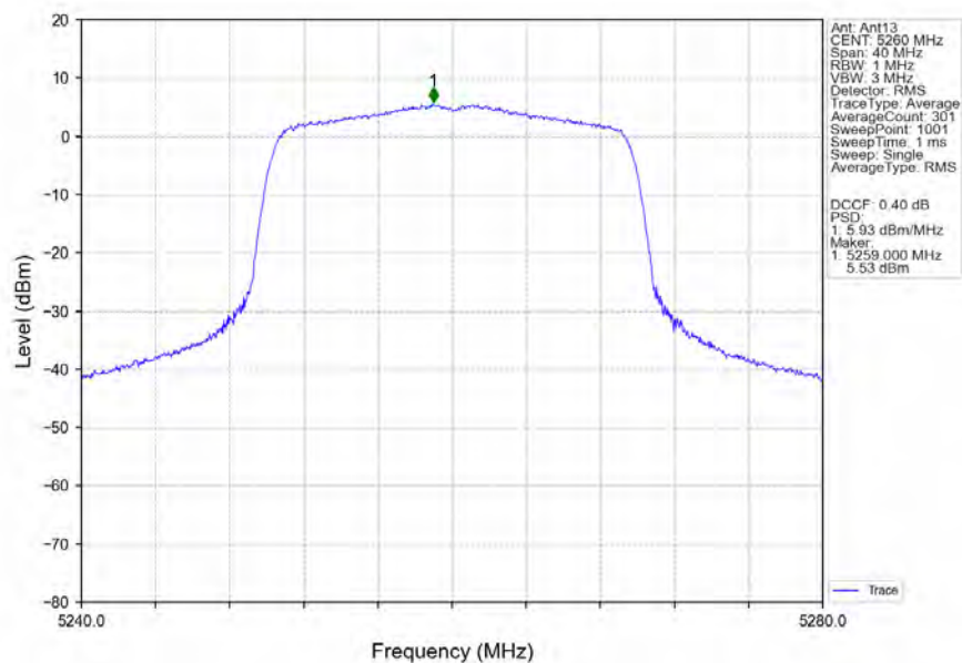
802.11ax(HEW20)_LCH_5260MHz_RU242_Left_Ant13_NTNV
