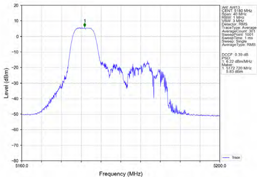
802.11ax(HEW20)_LCH_5180MHz_RU52_Left_Ant13_NTNV
