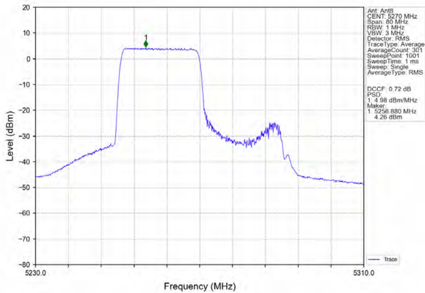
802.11ax(HEW40)_LCH_5270MHz_RU242_Left_Ant8_NTNV
