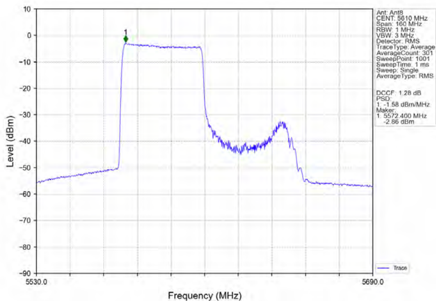
802.11ax(HEW80) HCH 5610MHz RU484 Right Ant8 NTN
