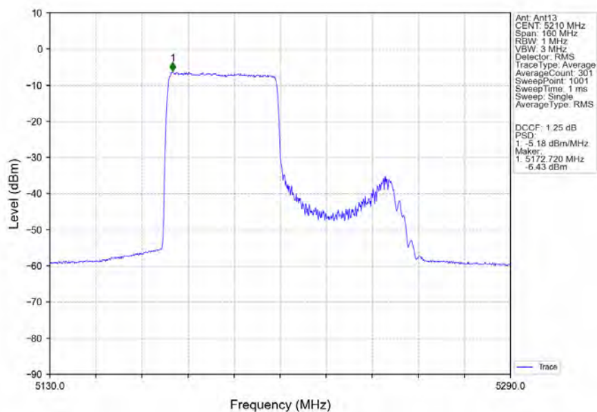
802.11ax(HEW80)_MCH_5210MHz_RU484_Left_MIMO_NTNV
