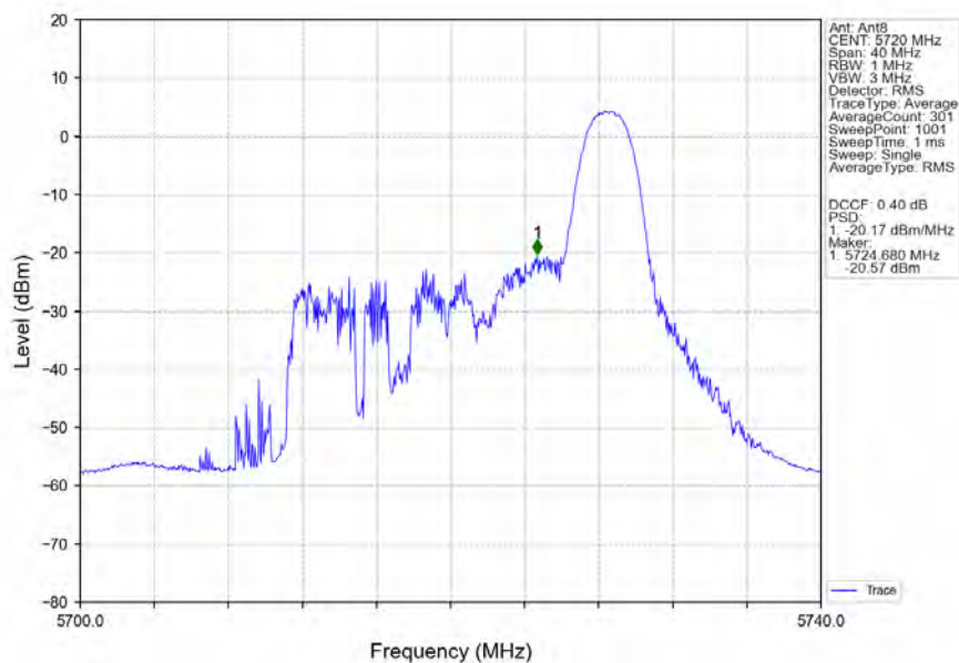
802.11ax(HEW20)_HCH_5720MHz_RU26_Right_Ant8_NTNV
