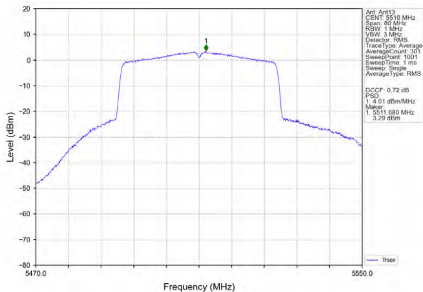
802.11ax(HEW40)_LCH_5510MHz_RU484_Left_Ant13_NTNV
