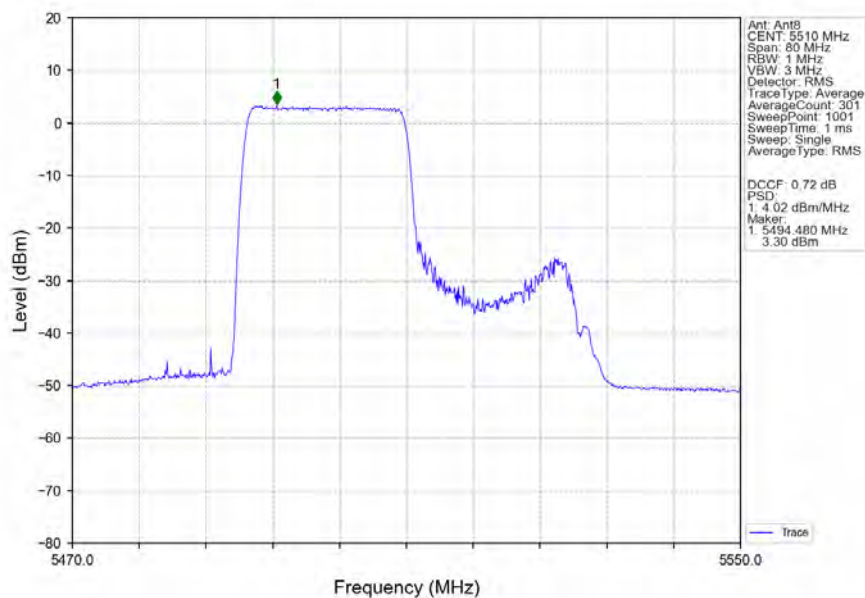
802.11ax(HEW40)_LCH_5510MHz_RU242_Left_Ant8_NTNV
