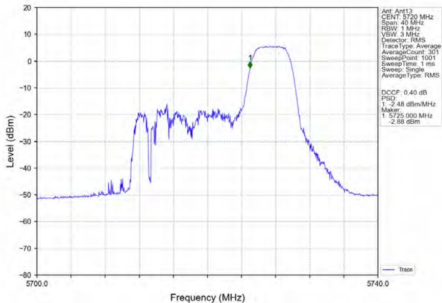
802.11ax(HEW20)_HCH_5720MHz_RU52_Right_Ant13_NTNV
