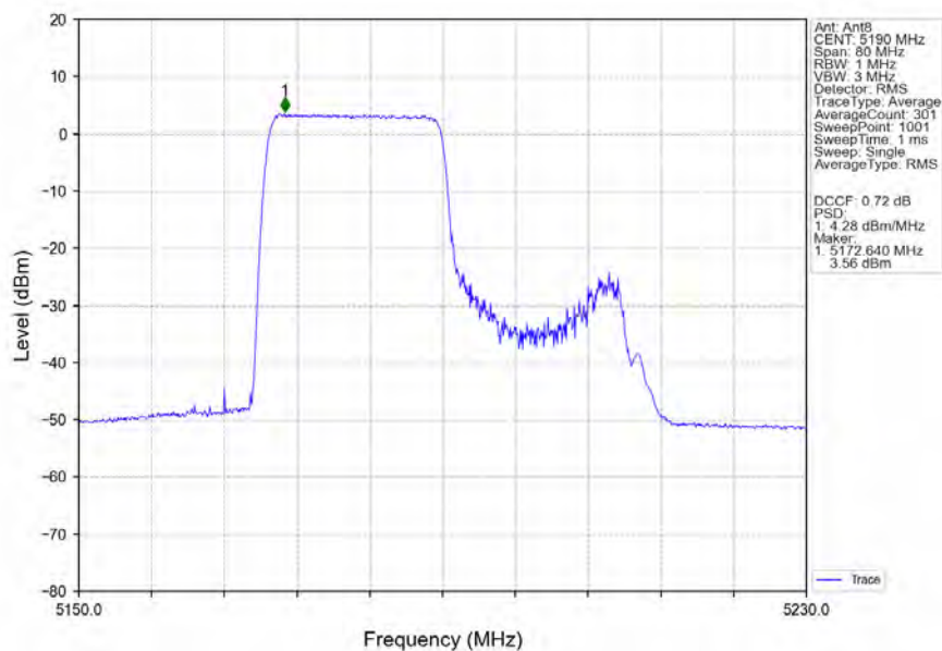
802.11ax(HEW40)_LCH_5190MHz_RU242_Left_Ant8_NTNV
