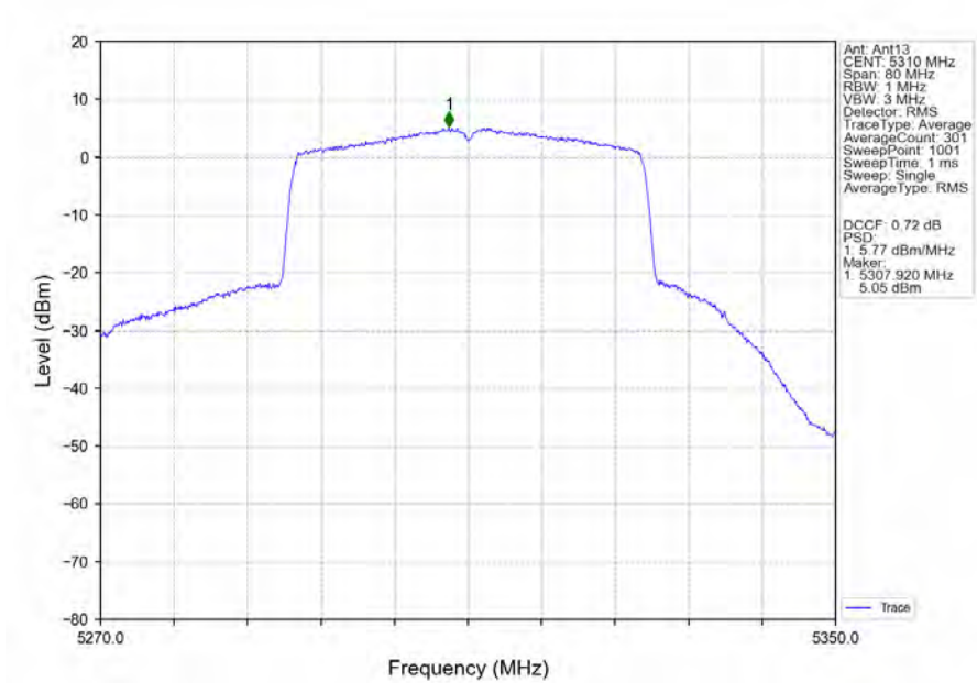
802.11ax(HEW40)_HCH_5310MHz_RU484_Left_Ant13_NTNV
