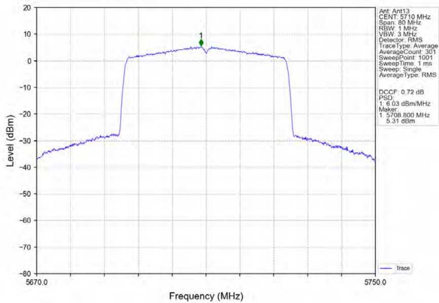
802.11ax(HEW40)_HCH_5710MHz_RU484_Left_Ant13_NTNV
