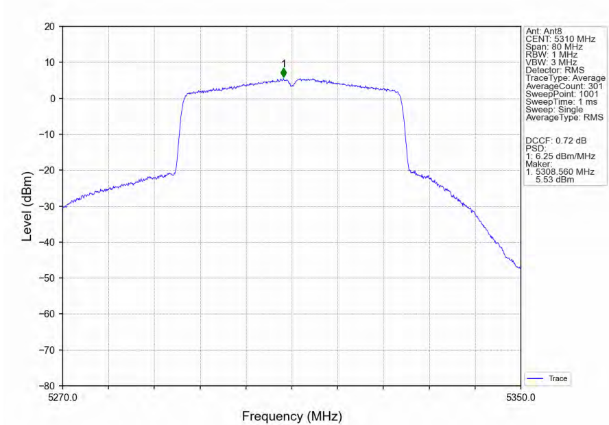
802.11ax(HEW40)_HCH_5310MHz_RU484_Left_Ant8_NTNV
