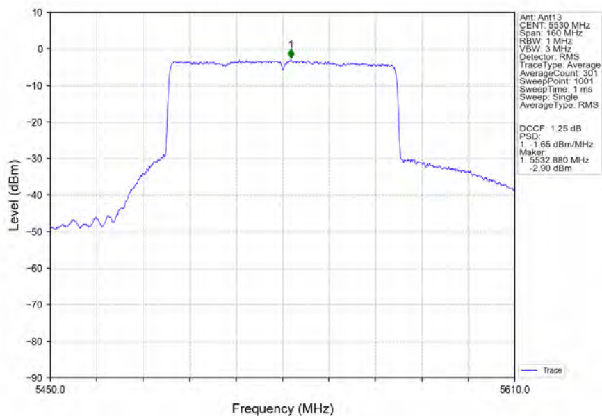
802.11ax(HEW80)_LCH_5530MHz_RU996_Left_Ant13_NTNV
