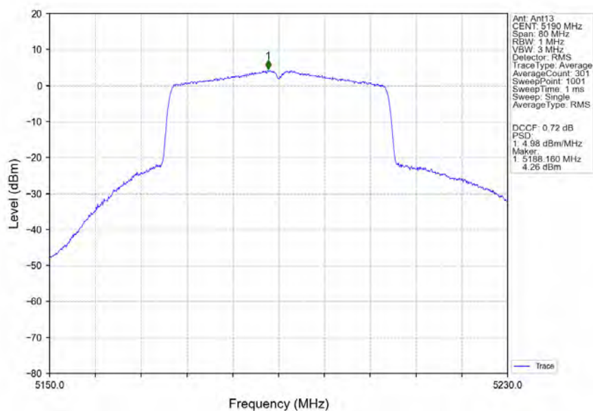
802.11ax(HEW40)_LCH_5190MHz_RU484_Left_Ant13_NTNV
