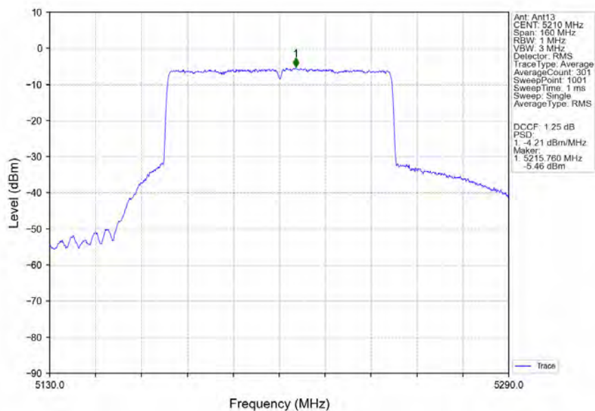
802.11ax(HEW80)_MCH_5210MHz_RU996_Left_Ant13_NTNV
