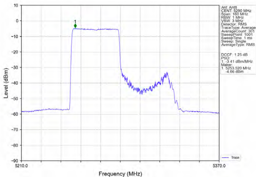
802.11ax(HEW80)_MCH_5290MHz_RU484_Left_Ant8_NTNV
