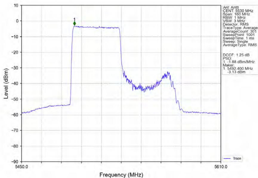
802.11ax(HEW80)_LCH_5530MHz_RU484_Left_Ant8_NTNV
