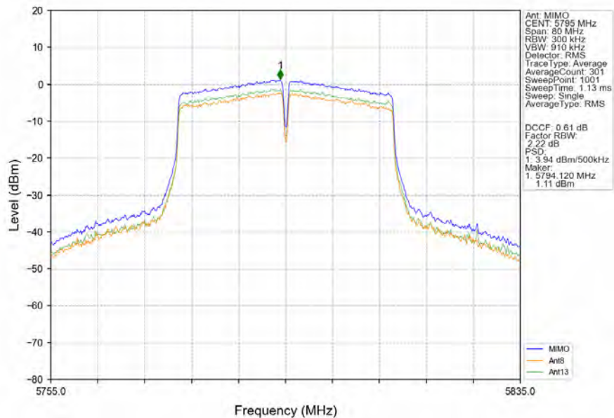
802.11n(HT40)_HCH_5795MHz_MIMO_NTNV
