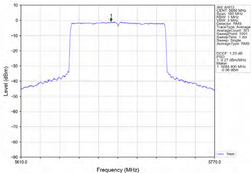
802.11ax(HEW80)_HCH_5690MHz_RU996_Left_Ant13_NTNV
