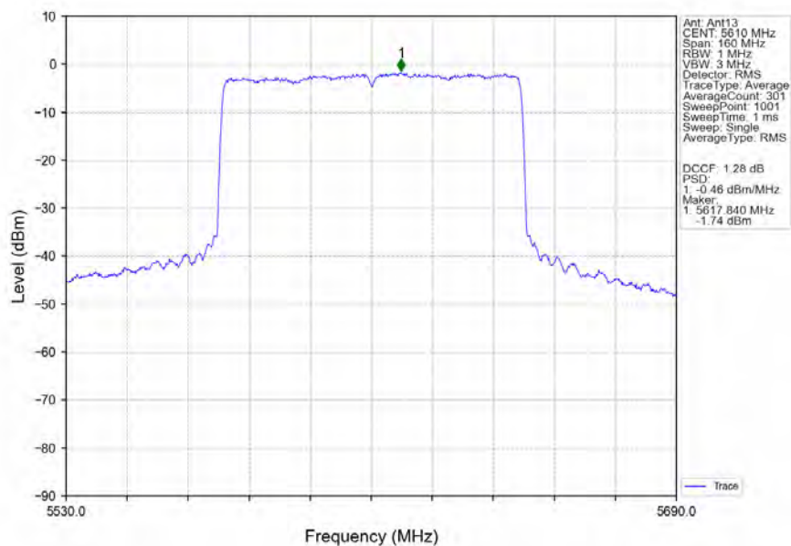
802.11ax(HEW80)_HCH_5610MHz_RU996_Left_Ant13_NTNV
