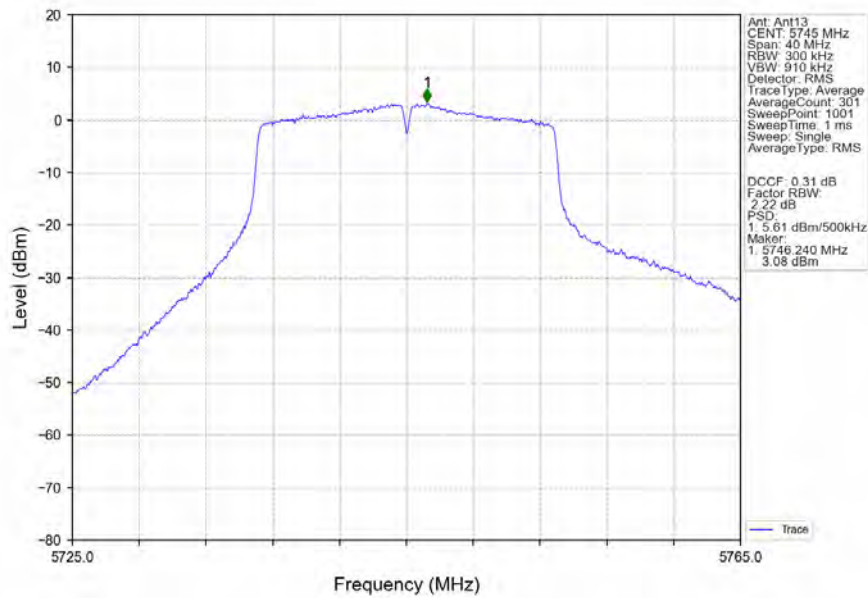
802.11n(HT20)_LCH_5745MHz_Ant13_NTNV
