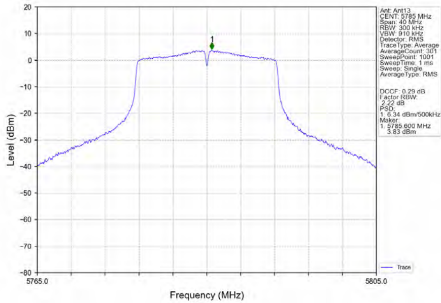
802.11a_MCH_5785MHz_MIMO_NTNV
