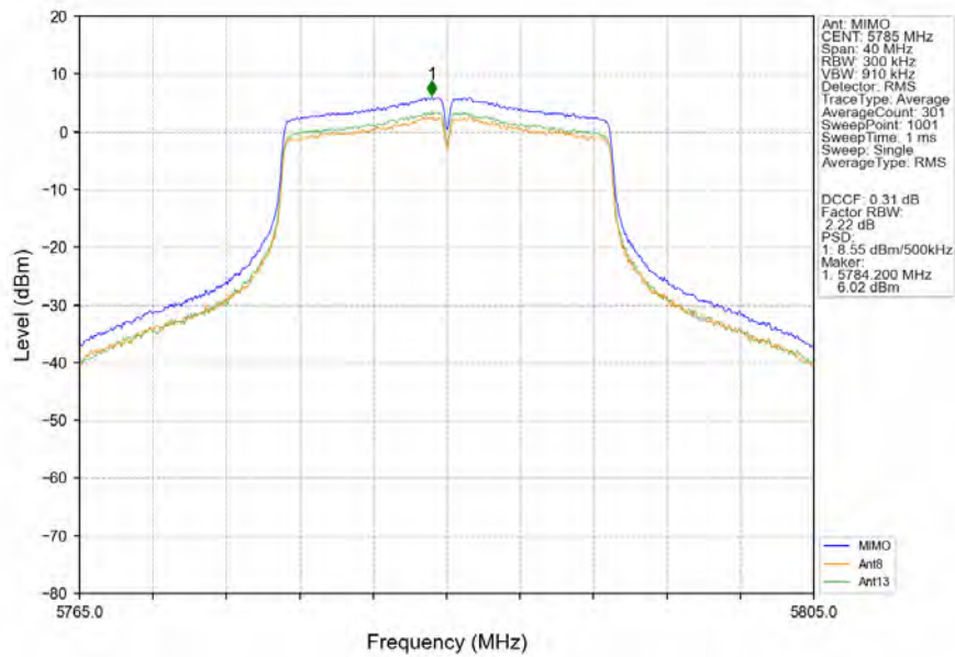
802.11n(HT20)_MCH_5785MHz_MIMO_NTNV
