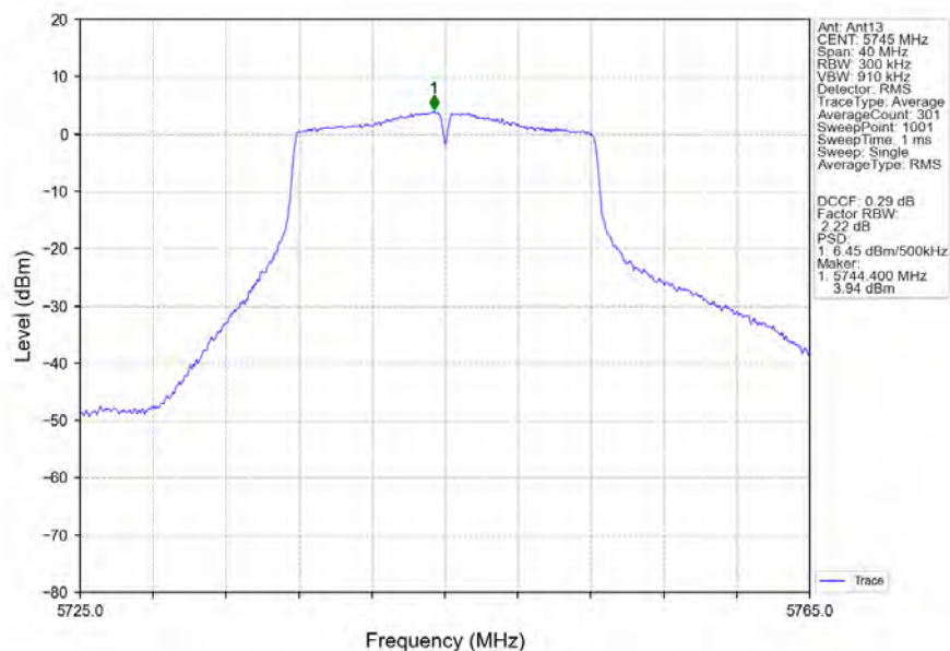
802.11a_LCH_5745MHz_Ant13_NTNV
