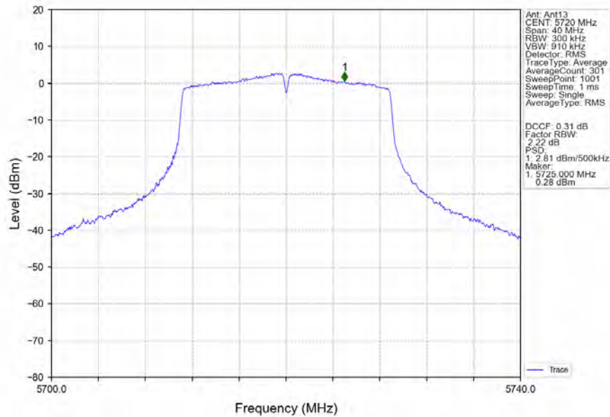
802.11n(HT20)_HCH_5720MHz_MIMO_NTNV
