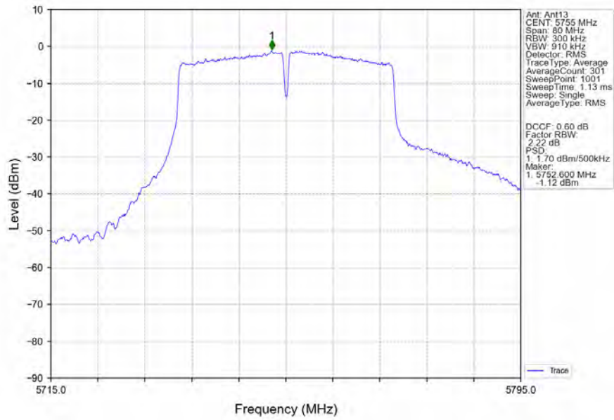
802.11ac(VHT40)_LCH_5755MHz_MIMO_NTNV
