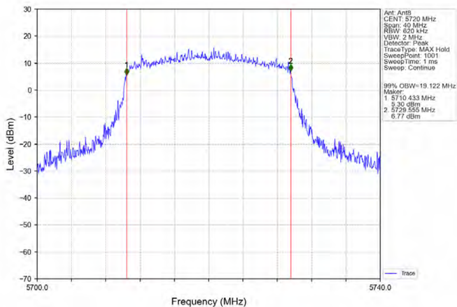
802.11ax(HEW20)_HCH_5720MHz_RU242_Left_Ant8_NTNV
