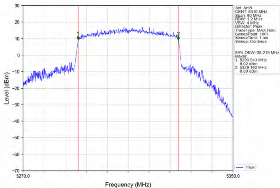
802.11ax(HEW40)_HCH_5310MHz_RU484_Left_Ant8_NTNV
