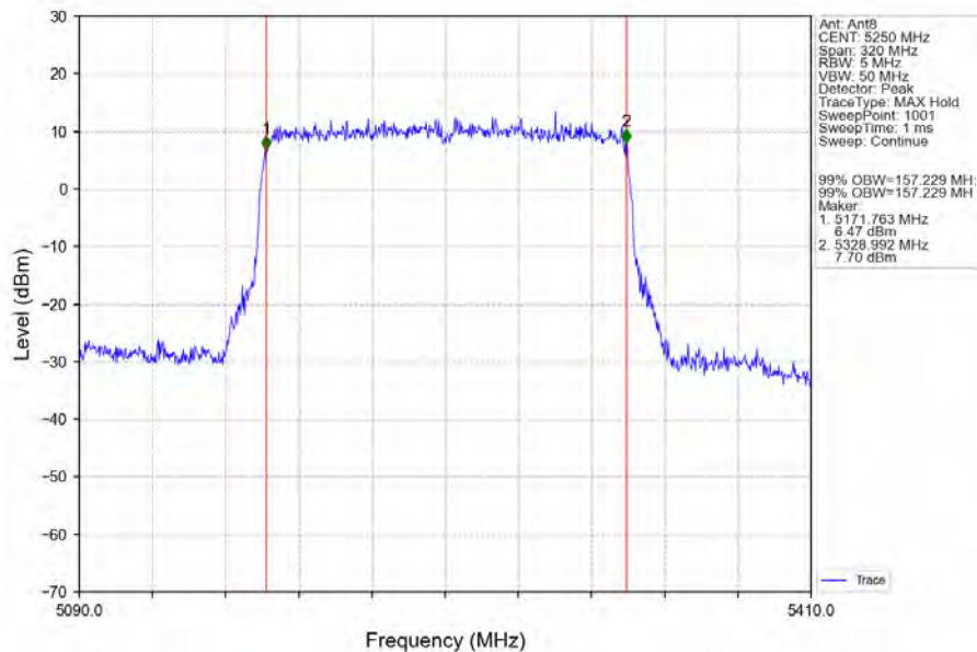
802.11ax(HEW160) MCH_5250MHz_2xRU996_Left_Ant8_NTNV
