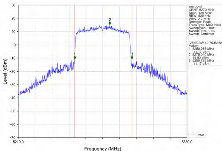
802.11ax(HEW40)_LCH_5270MHz_RU484_Left_Ant8_NTNV
