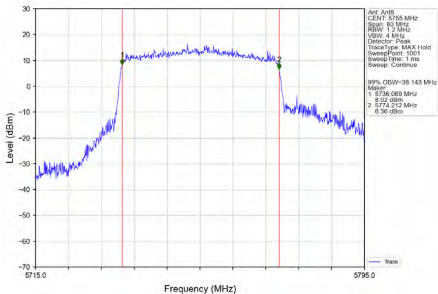
802.11ax(HEW40)_LCH_5755MHz_RU484_Left_Ant8_NTNV
