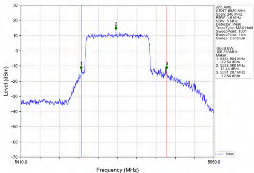
802.11ax(HEW80)_LCH_5530MHz_RU996_Left_Ant8_NTNV
