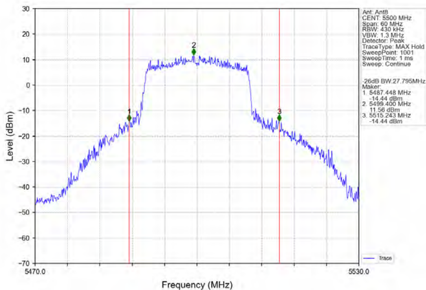
802.11ax(HEW20)_LCH_5500MHz_RU242_Left_Ant8_NTNV
