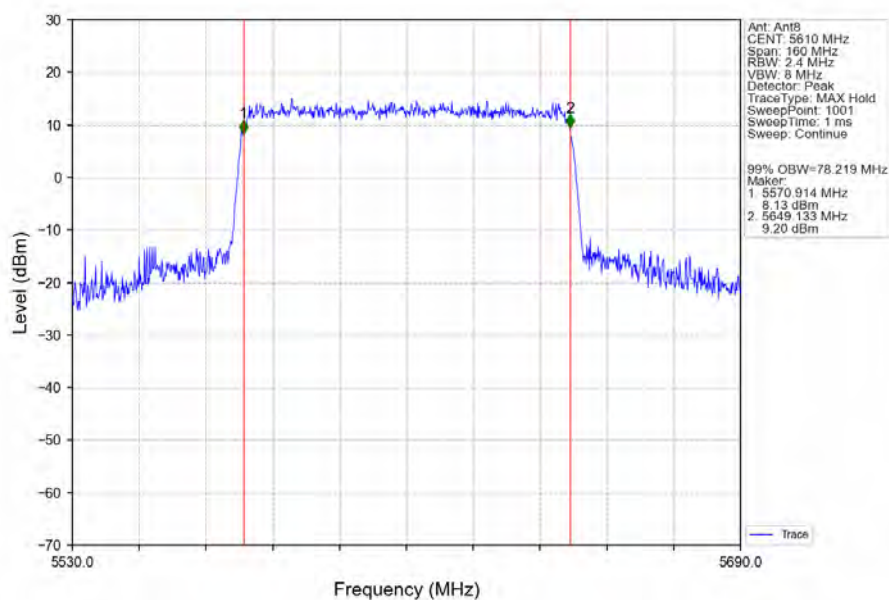
802.11ax(HEW80)_HCH_5610MHz_RU996_Left_Ant8_NTNV
