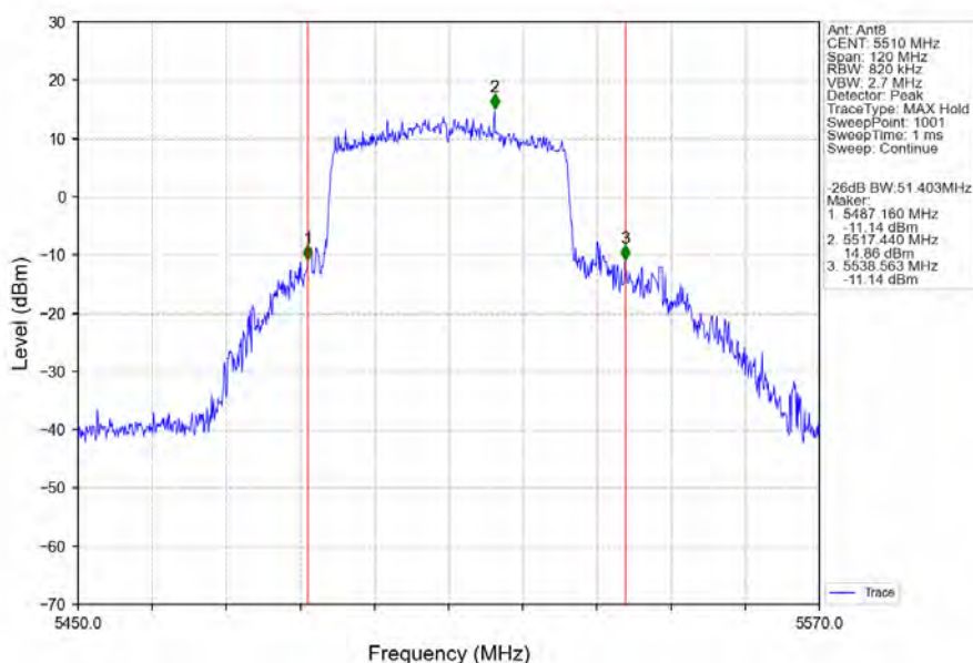
802.11ax(HEW40)_LCH_5510MHz_RU484_Left_Ant8_NTNV
