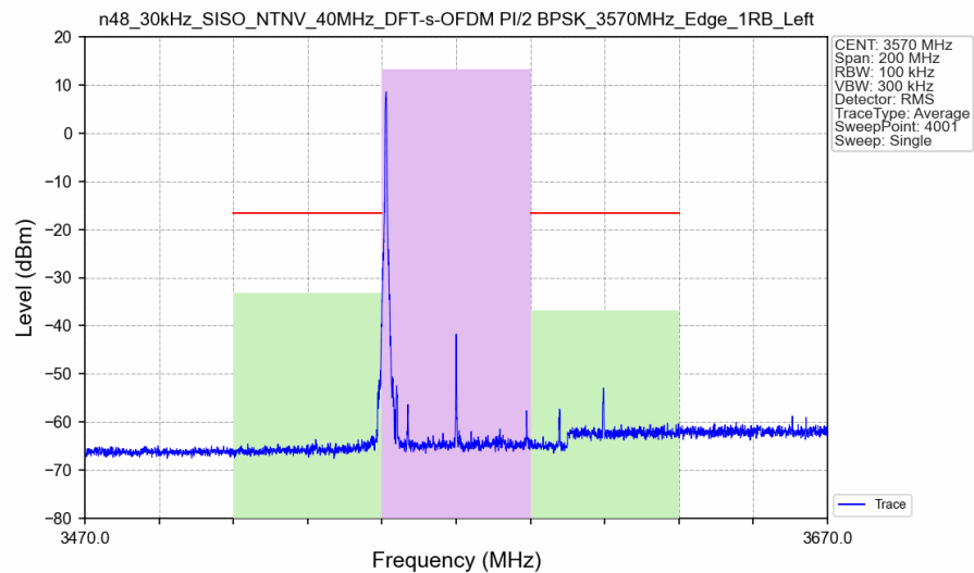
n48_30kHz_SISO_NTNV_40MHz_DFT-s-OFDM PI/2 BPSK_3570MHz_Edge_1RB_Left_Ant8
