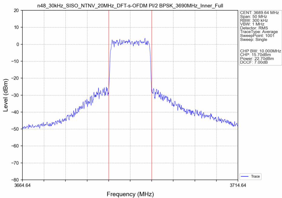
n48_30kHz_SISO_NTNV_20MHz_DFT-s-OFDM PI/2 BPSK_3690MHz_Inner_Full_Ant8
