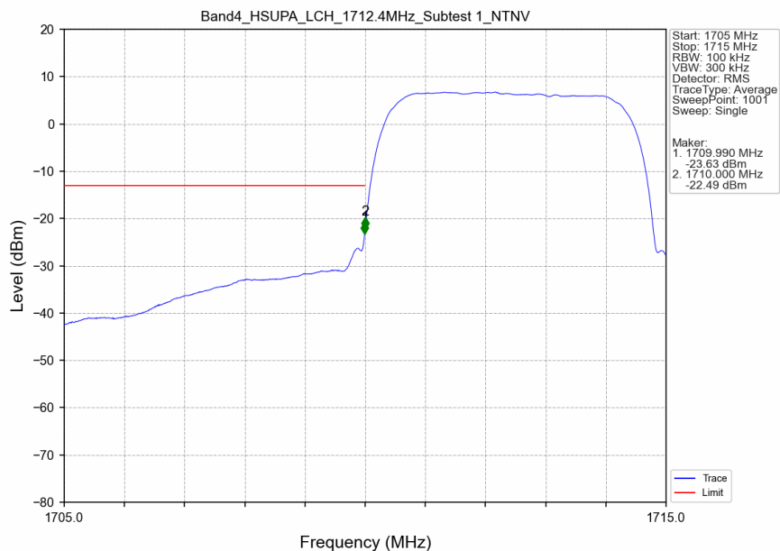
Band4_HSUPA_LCH_1712.4MHz_Subtest 1_NTNV
