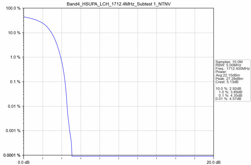
Band4_HSUPA_LCH_1712.4MHz_Subtest 1_NTNV
